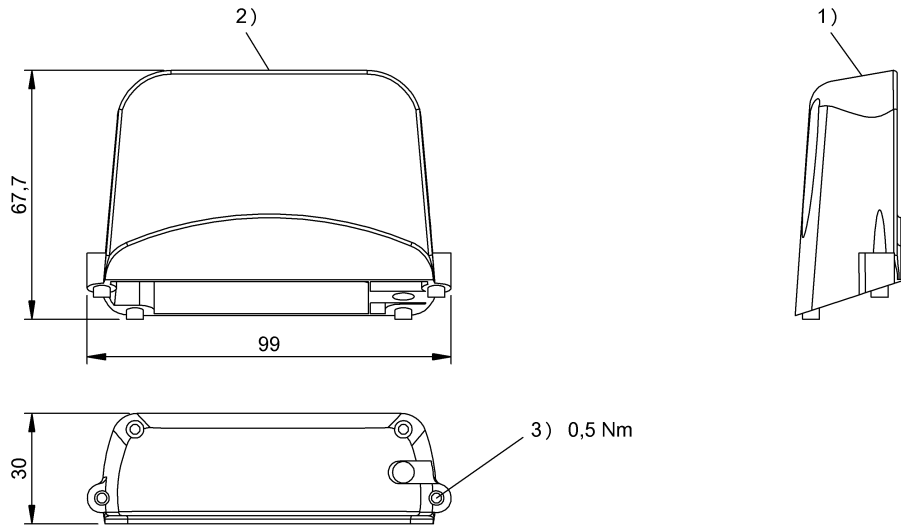
1) Активная поверхность 2) Форму антенны см. в данных 3) Момент затяжки
