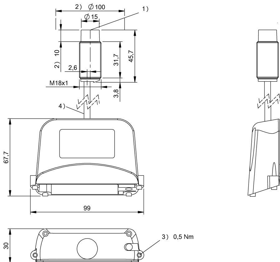
1) Активная поверхность 2) Свободная зона 3) Момент затяжки 4) Длину кабеля см. в тексте
