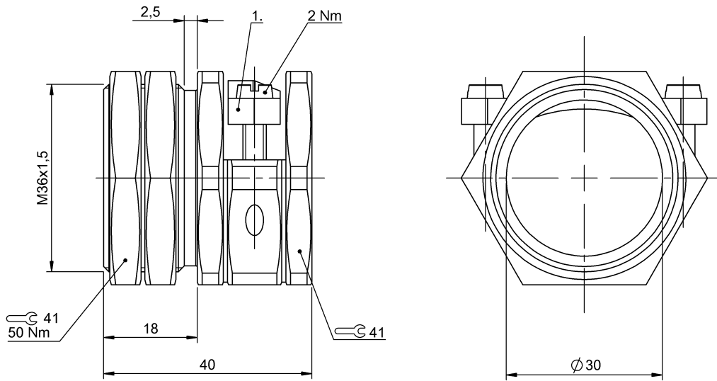
1) Зажимная скоба
