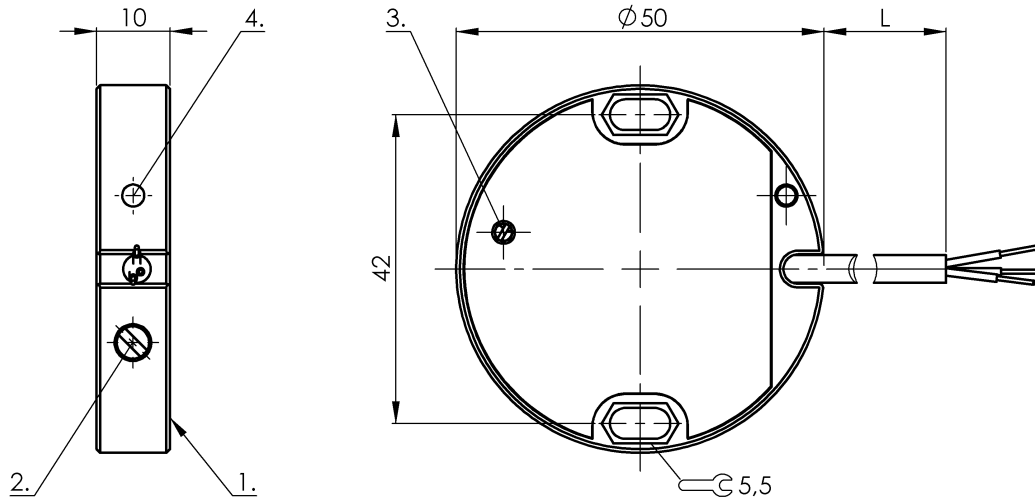
1) Активная поверхность 2) Потенциометр 3) По выбору замыкатель или размыкатель 4) Функциональный СИД
