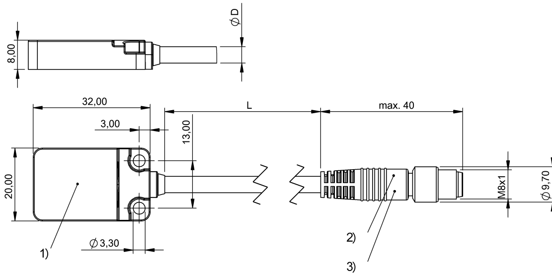
1) Активная поверхность 2) СИД желтый 3) СИД зеленый
