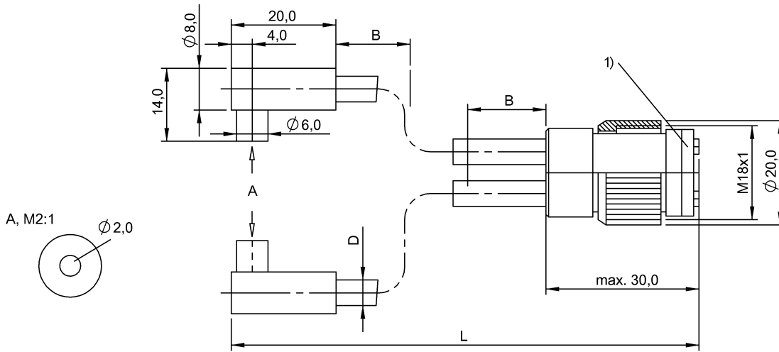
1) Съемная шайба
