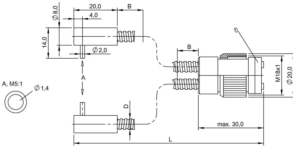
1) Съемная шайба
