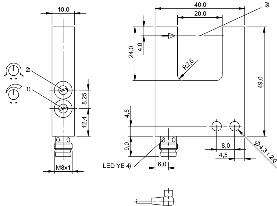
1) Чувствительность 2) Включение при освещении / затемнении 3) Оптическая ось 4) Функция выхода
