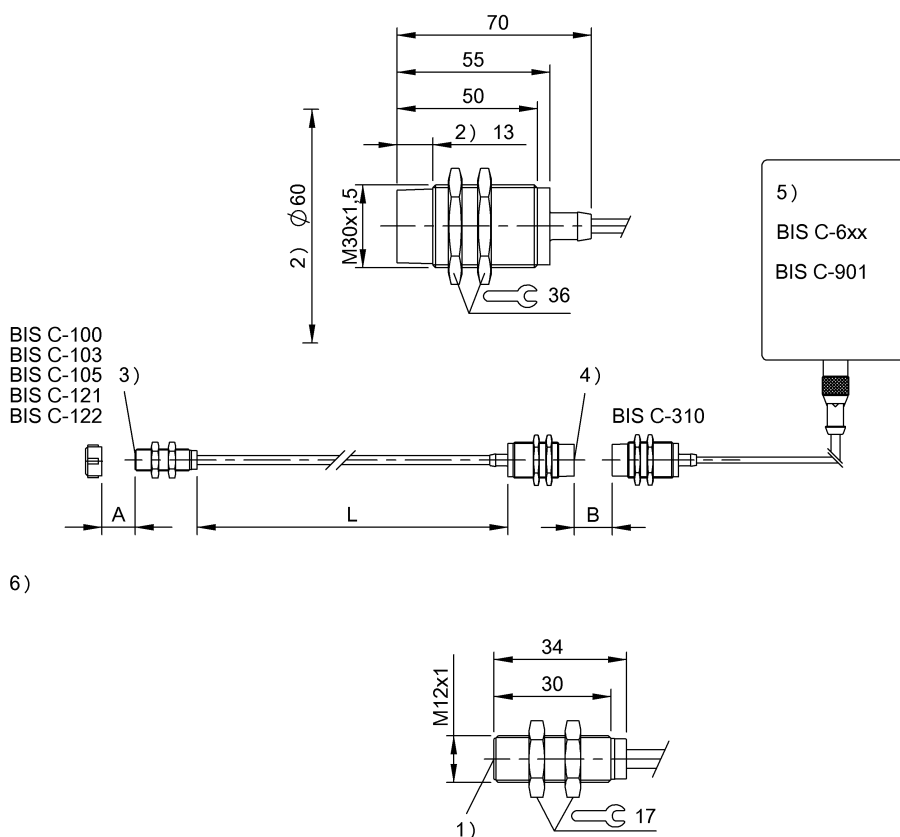
1) Активная поверхность 2) Свободная зона 3) Активная поверхность носителя данных 4) Активная поверхность головки зап./счит. 5) Блок обработки результатов или преобразователь 6) См. примечания
