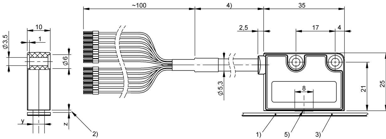
1) Не входит в комплект поставки 2) Расстояние до мерной ленты 3) Мерный объект 4) Длина кабеля 5) активная измер. поверхность
