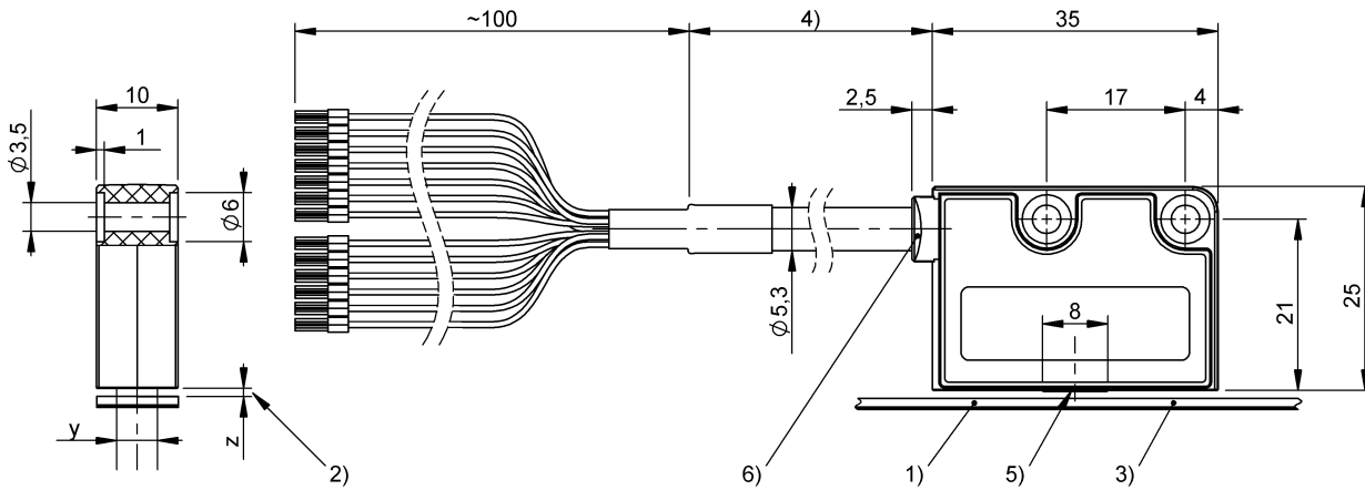
1) Не входит в комплект поставки 2) Расстояние до мерной ленты 3) Мерный объект 4) Длина кабеля 5) активная измер. поверхность 6) СИД сигнализации сбоев
