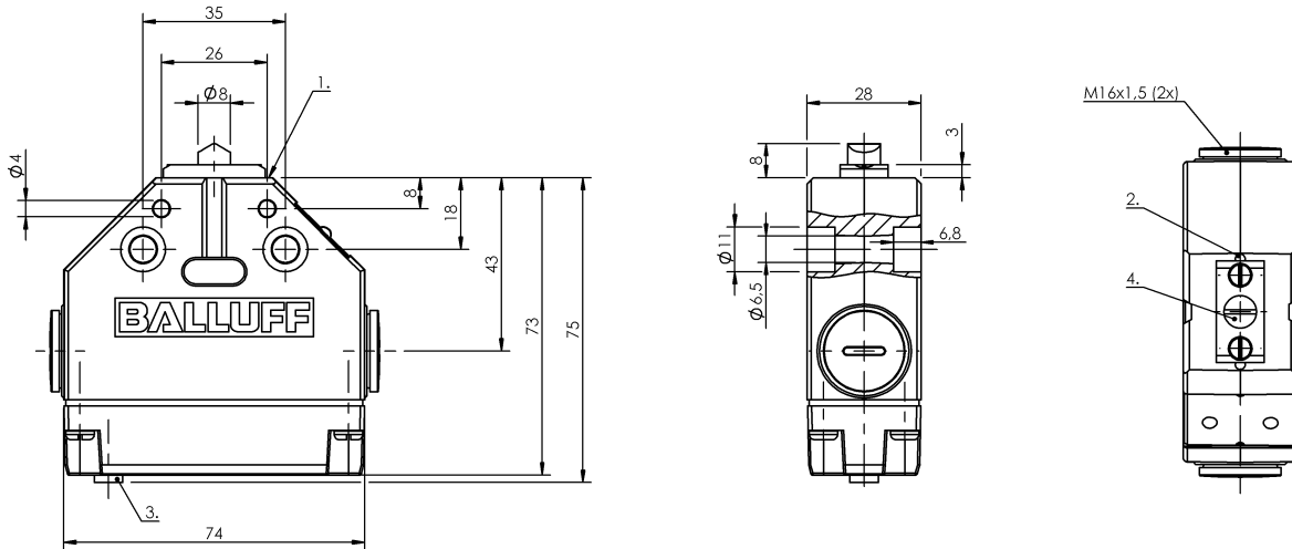
1) Опорная кромка 2) Марк. Предохран. точка коммутации 3) Функциональный индикатор FC 4) Противокристаллизационный толкатель
