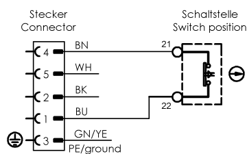
PE mit Gehäuse verbunden ground connected to housing
