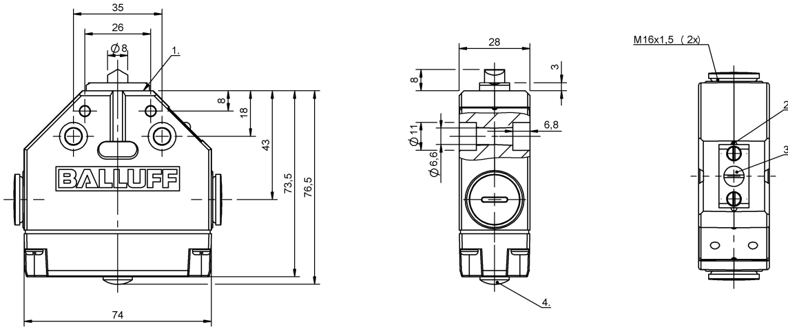
1) Опорная кромка 2) Марк. Предохран. точка коммутации 3) Противокристаллизационный толкатель 4) Функциональный индикатор FD/FE/LL
