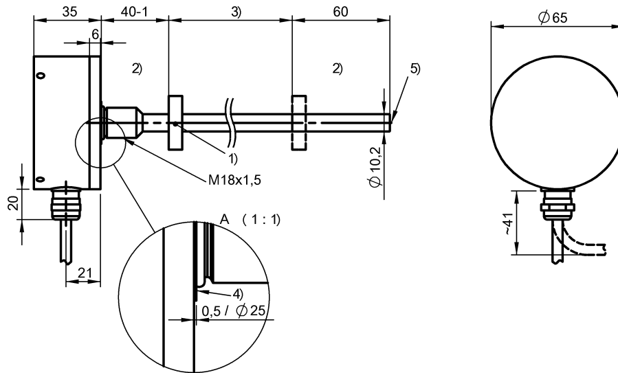
1) Не входит в комплект поставки 2) неиспользуемая область 3) Номинальная длина = измеряемая длина 4) Контактная поверхность 5) Внутренняя резьба M4x4/6 глубокая
