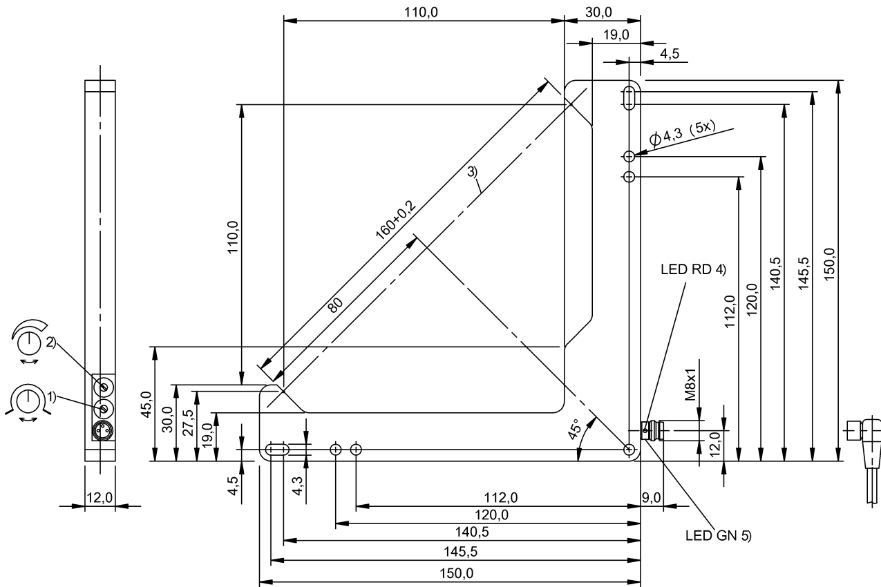
1) Включение при освещении / затемнении 2) Чувствительность 3) Оптическая ось 4) Функция выхода 5) Напряжение питания
