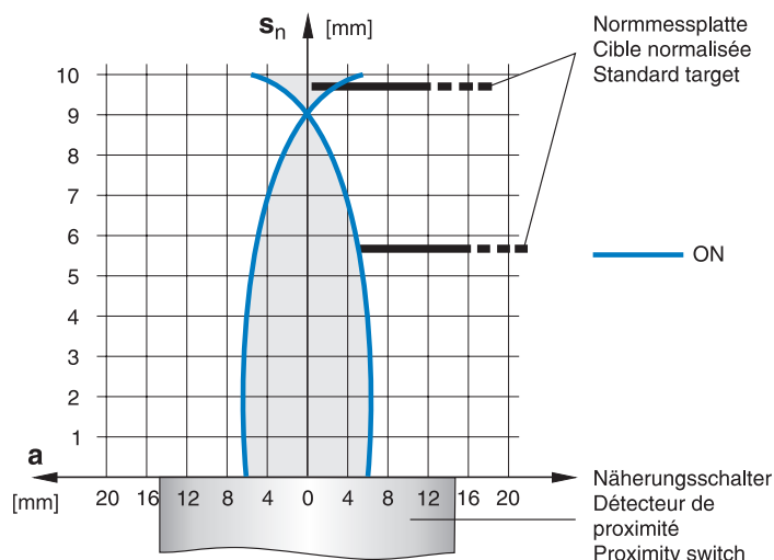
DW-AD-70#-M30-BAS
