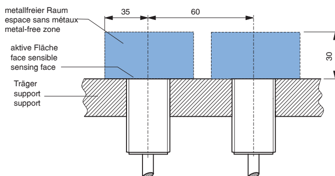
DW-AS-70#-M30-BAS
