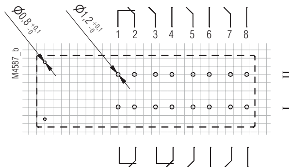
OA5623.58/___W1 5NO/3NC
