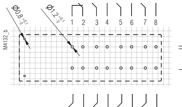
OA5623.63/___W5 7NO/1NC
