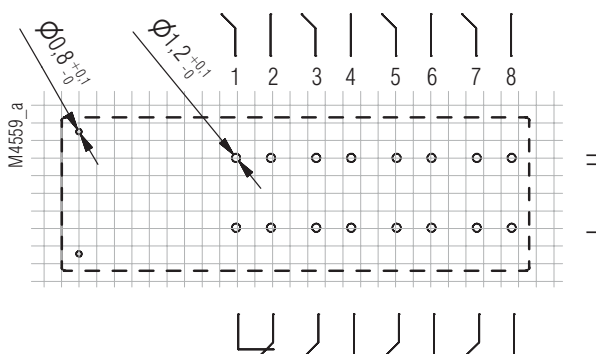
OA5623.63/___W1 7NO/1NC
