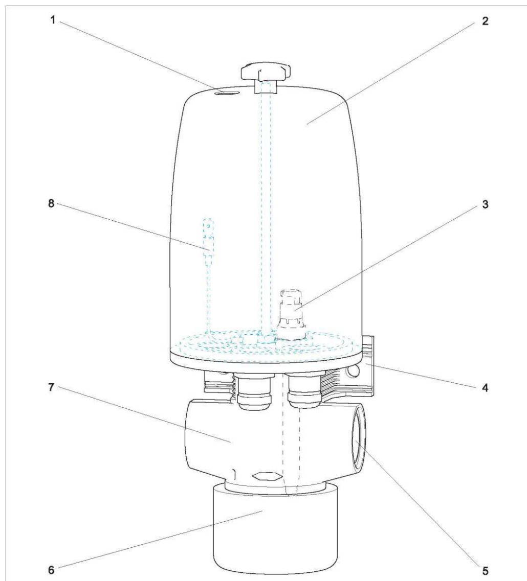
Рис. 1. Арматура SPA250 с датчиком
