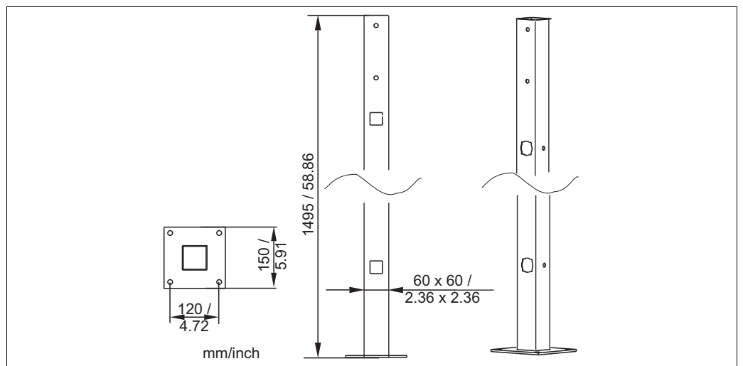
Fig. 50: Universal post
