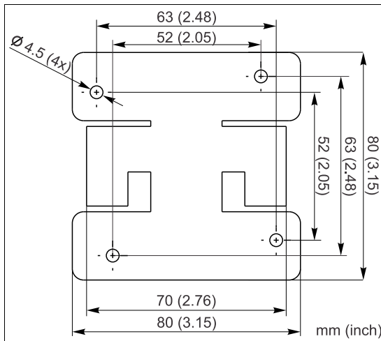
Maße Befestigungsplatte
