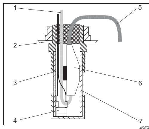
Fig. 11: Pipe socket
