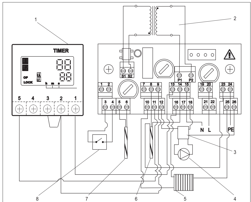
Fig. 13: Wiring diagram
