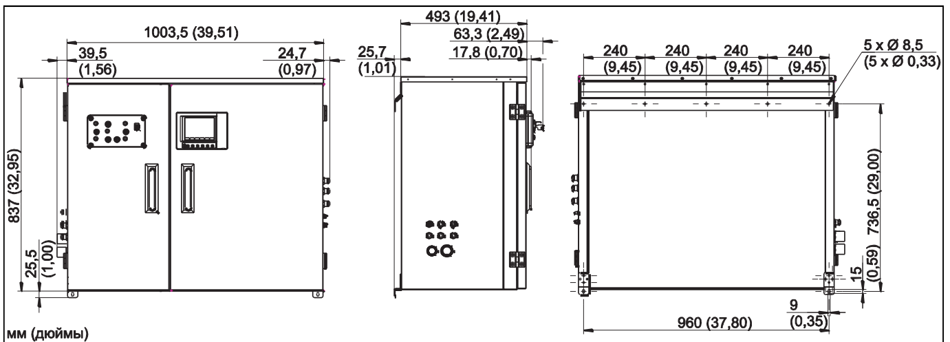
Размеры корпуса СУС310, исполнение из нержавеющей стали
