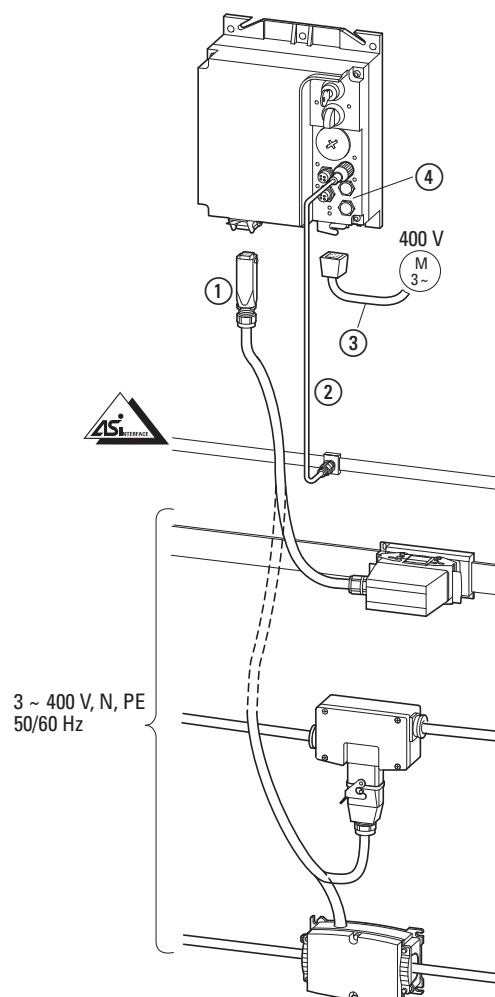
Figure 80 : Raccordements sur le module RAMO
