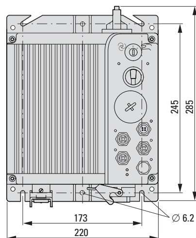
Figure 122: RASP-2, RASP-3, RASP-4 avec interrupteur de maintenance
