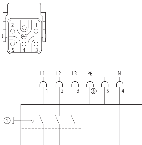
Figure 7 : Interrupteur de maintenance en position 0 = arrêt
