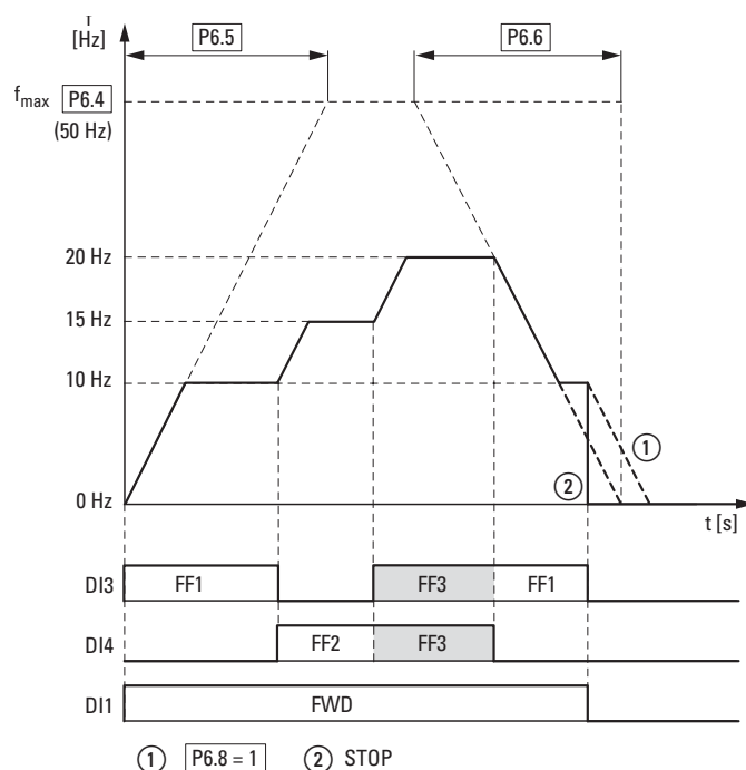
Figure 109: Exemple : activation des fréquences présélectionnées, avec rampes d'accélération et de décélération DQ2 → DI3 = FF1 (P10.2) DQ3 → DI4 = FF2 (P10.3) DQ2 + DQ3 → DI3 + DI4 = FF1 FF3 (P10.2)
