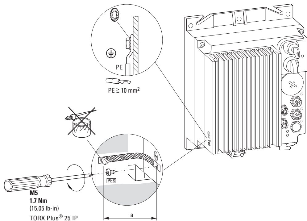
Figure 61 : Mise à la terre fonctionnelle (toron ou câble rond)
