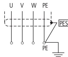
Figure 58 : Raccordement de la tresse blindée (PES) sur le bornier moteur
