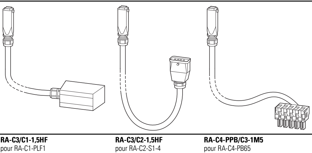
Figure 50 : Connecteur d'alimentation avec câble adaptateur (Eaton)
