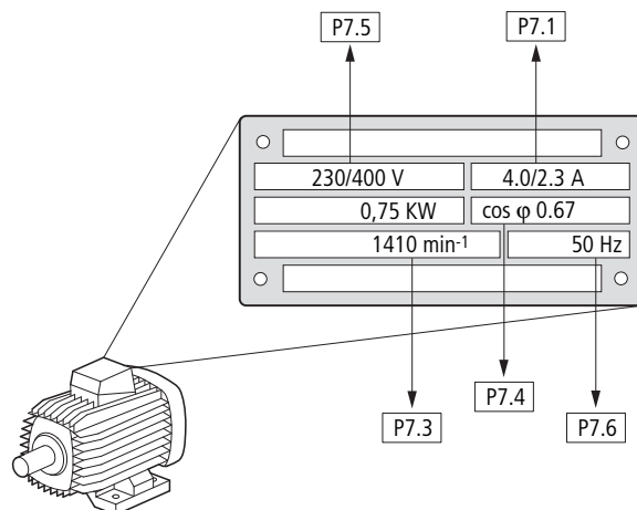
Figure 107: Paramètres moteur indiqués sur la plaque signalétique
