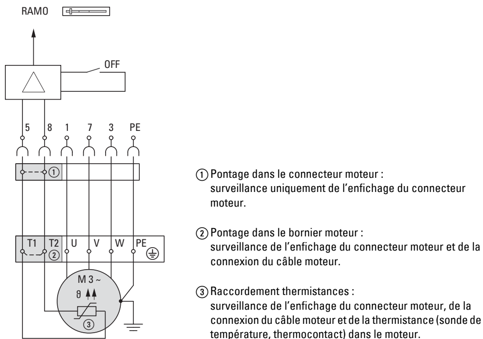
Figure 27 : Surveillance par codeur DIP et pressostat
