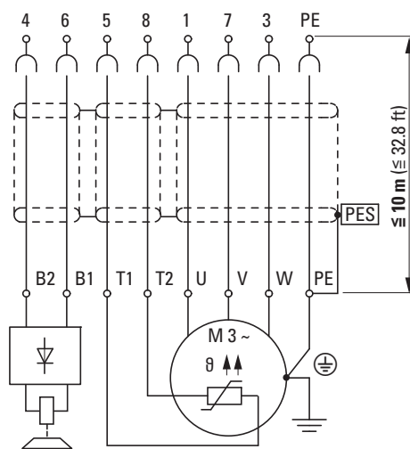
Figure 55 : Câble moteur blindé avec module RASP. Longueur max. admissible du câble moteur : 10 m
