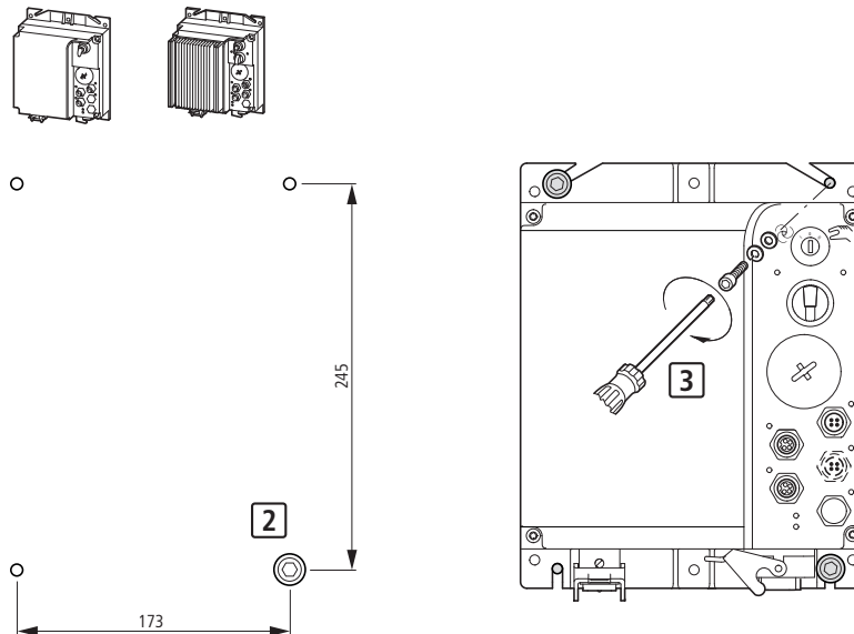
Figure 31 : Cotes de fixation (standard) et montage
