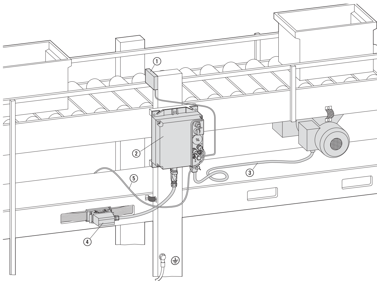
Figure 6 : Exemple de montage d'un module RAMO
