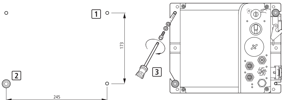
Figure 33 : Cotes de fixation (standard) et montage
