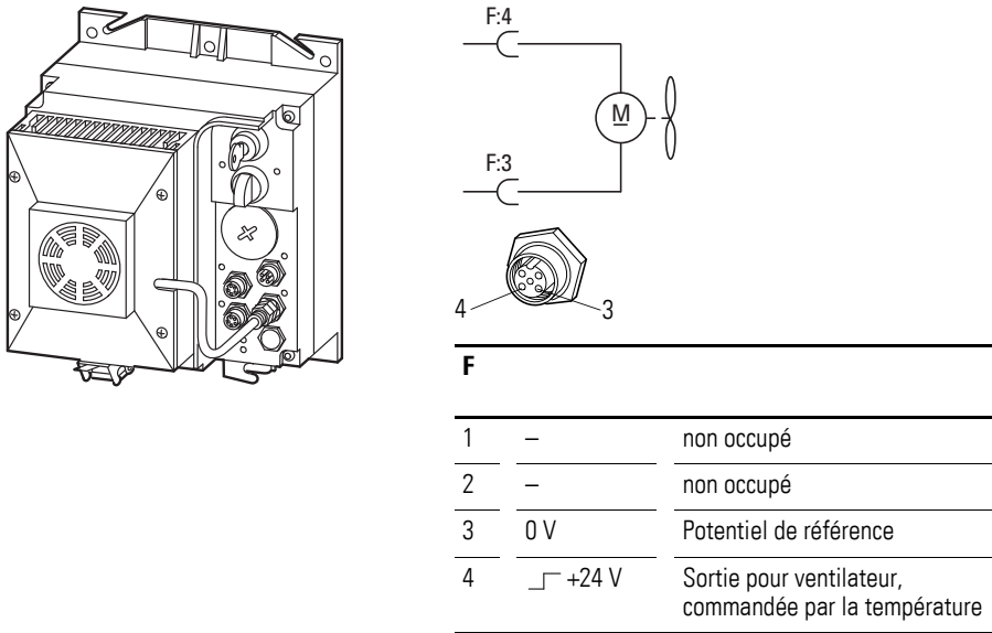
Figure 19 :Raccordement de ventilateur F
