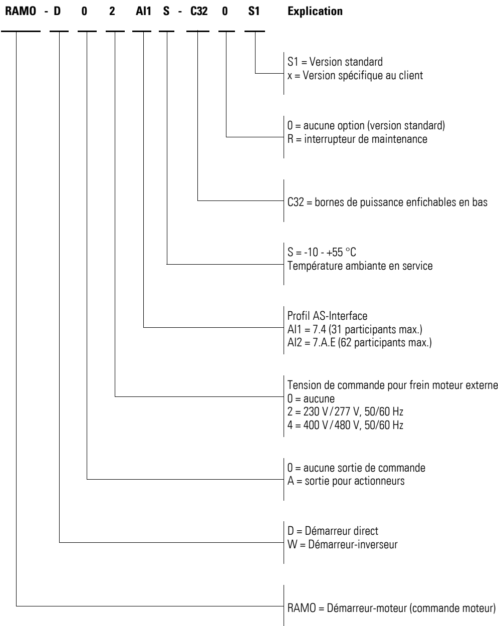
Figure 3 : Signification des références du démarreur-moteur RAMO
