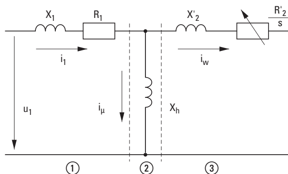
Figure 112 :Schéma équivalent de moteur asynchrone triphasé
