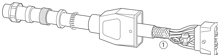
Figure 60 : Câble moteur avec mise à la terre Δ PES
