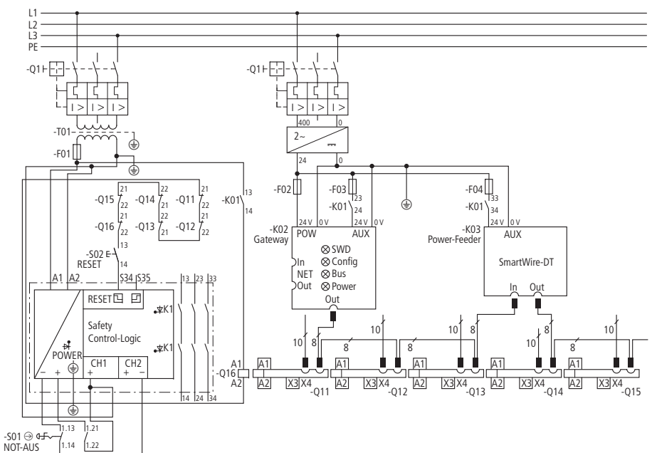
Abbildung 48: Stromkreis für redundante Abschaltung von Antriebsgruppen
