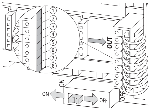
Abbildung 75: Abschlusswiderstand
