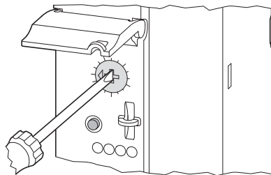
Abbildung 64: Motorstrom einstellen
