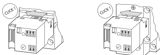
Abbildung 35: Verriegeln des DIL-SWD-32-001 bzw. des DIL-SWD-32-002
