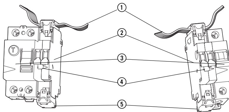
Abbildung 84: Aufbau MCB-HK-SWD
