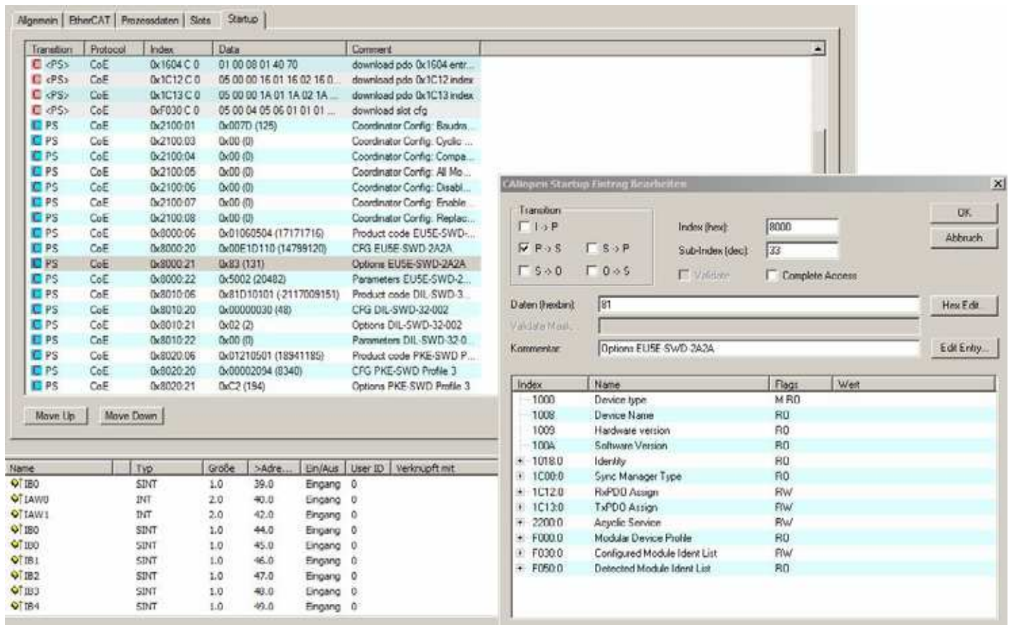
Abbildung 97: Ändern des Optionsbytes beim Modul EU5E-SWD-2A2A
