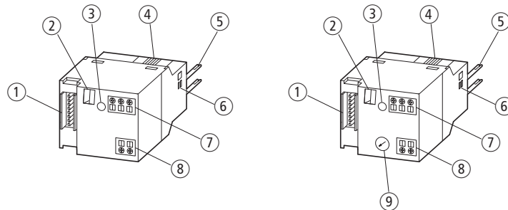
Abbildung 24: Aufbau der SmartWire-DT Module DIL-SWD-32-001 und DIL-SWD-32-002 für DILM
