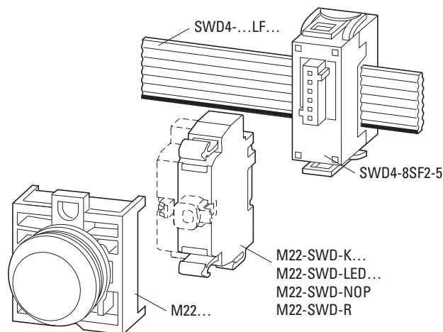
Abbildung 65: Aufbau M22-SWD-Frontbefestigung
