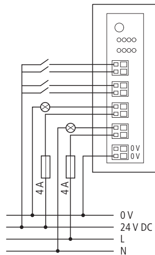
Abbildung 15: Anschluss der Ein-/Ausgänge des Moduls EU5E-SWD-4D2R
