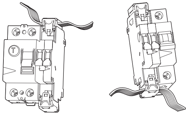
Abbildung 87: Anschluss der SmartWire-DT Leitung
