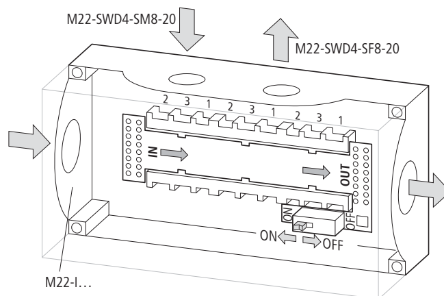
Abbildung 74: Aufbaugehäuse mit Leiterplatte M22-SWD-ILP...
