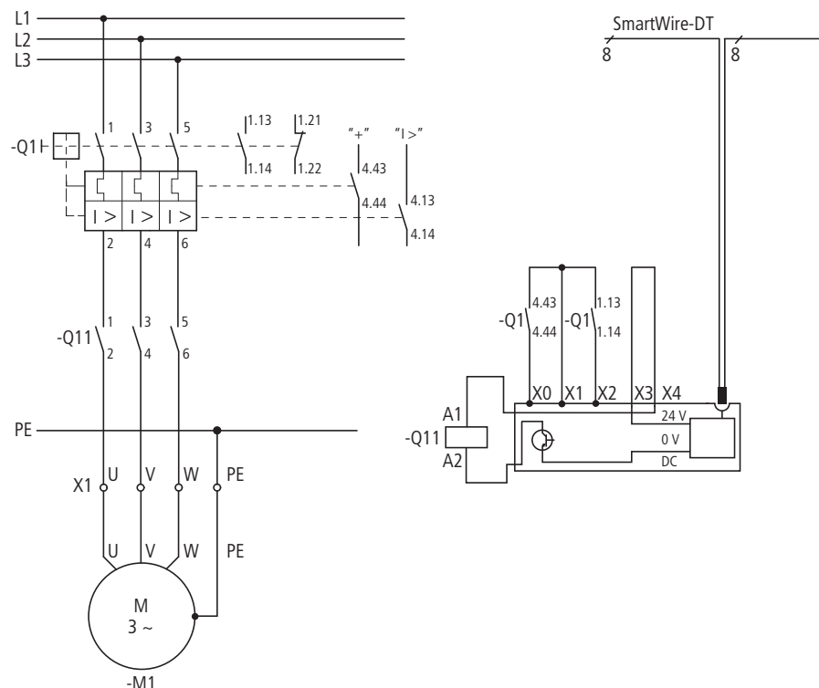
Abbildung 26: Stromlaufplan des Direktstarters
