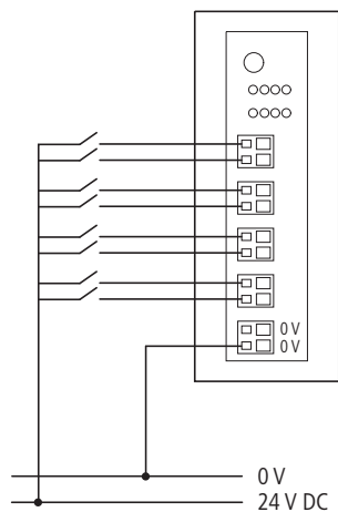
Abbildung 9: Anschluss der Eingänge und des Bezugspotenzials
