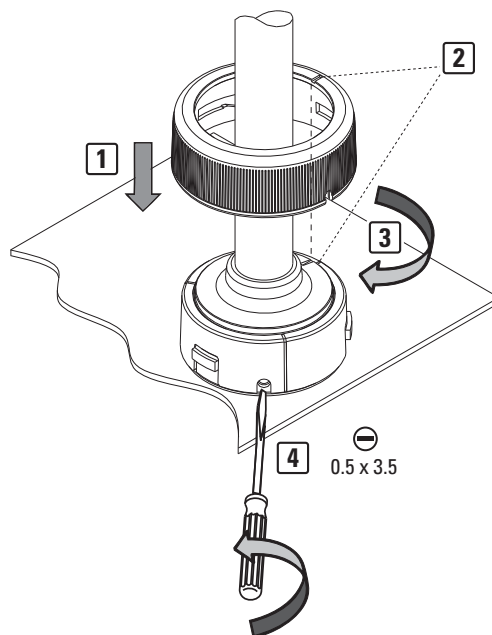
Abbildung 80: Befestigen des Basismoduls auf dem Schnellmontageadapter
