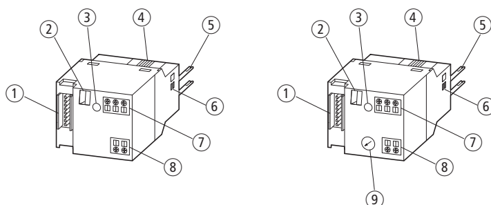
Abbildung 25: Anschlüsse des SmartWire-DT Moduls DIL-SWD-32-001 bzw. DIL-SWD-32-002 für DILM
