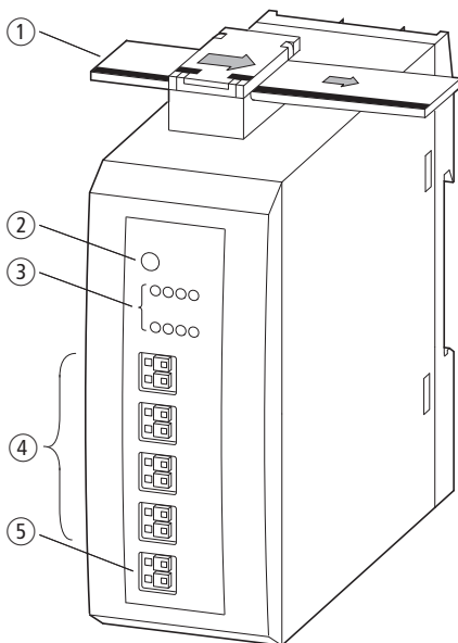
Figura 12: Collegamenti del modulo SWD I/O
