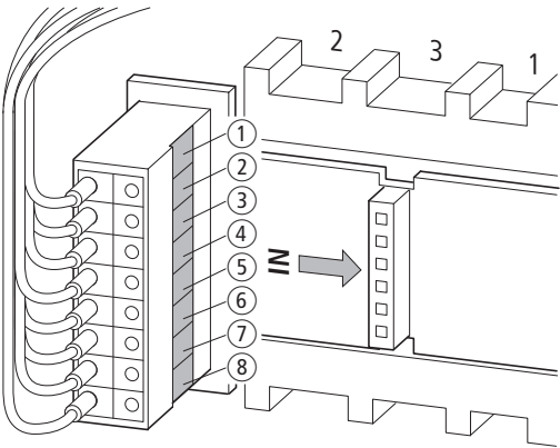
Figura 23: Modulo con morsettiera con collegamento in ingresso (IN)
