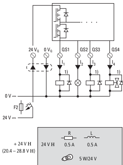
Figura 18: Uscite transistor ES4P-22-DM.. 1) Utilizzare diodi soppressori per apparecchi ES4P-221-DMX.. di versione 02 e 10
