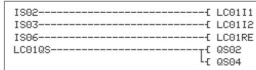
Figura 206: Esempio 2 "Griglia ottica" : schema elettrico in easySafety
