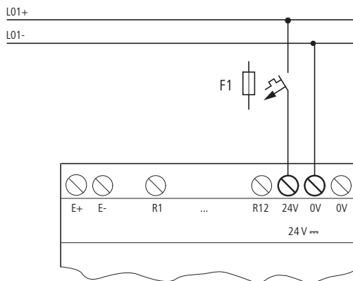
Figura 9: Tensione di alimentazione per l'apparecchio di espansione DC
