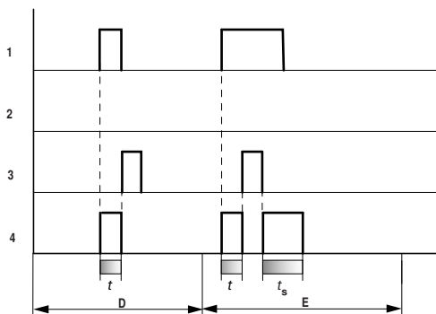
Figura 163: Diagramma di stato temporizzatore, a generazione di impulsi 2
