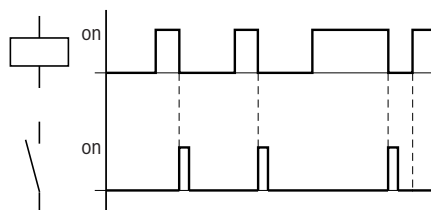
Figura 64: Diagramma di stato "impulso di ciclo" con fronte negativo
