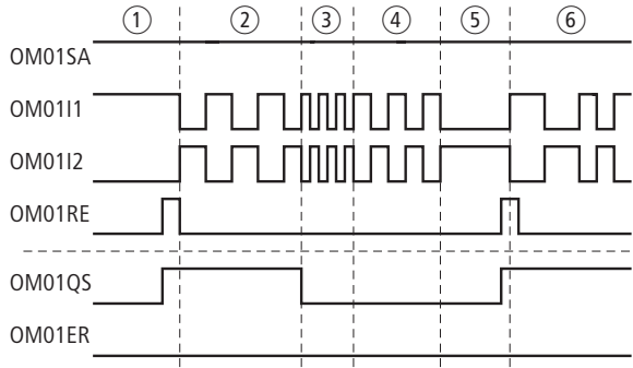
Figura 226: Esempio "Monitoraggio del numero di giri massimo": diagramma temporale
