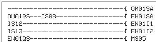
Figura 183: Esempio "Interruttore di approvazione": schema elettrico in easySafety
