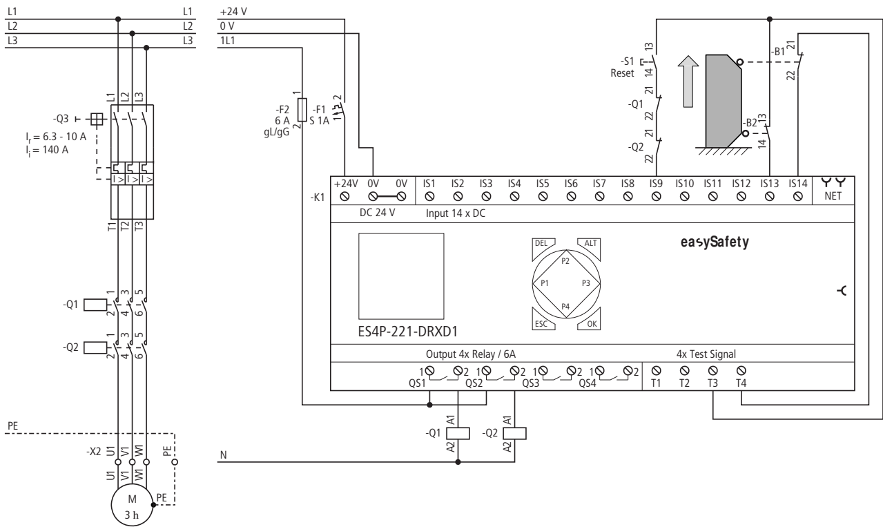
Figura 242: Esempio 1 "Porta di sicurezza": schema elettrico
