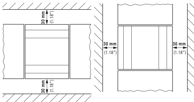
Figura 4: Distanze dall'apparecchio easySafety
