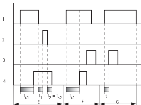
Figura 160: Diagramma di stato temporizzatore, ritardato all'eccitazione e alla diseccitazione 2
