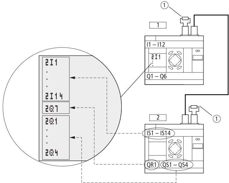
Figura 283: Usare gli ingressi e le uscite di un apparecchio easySafety nello schema elettrico standard di un altro utente
