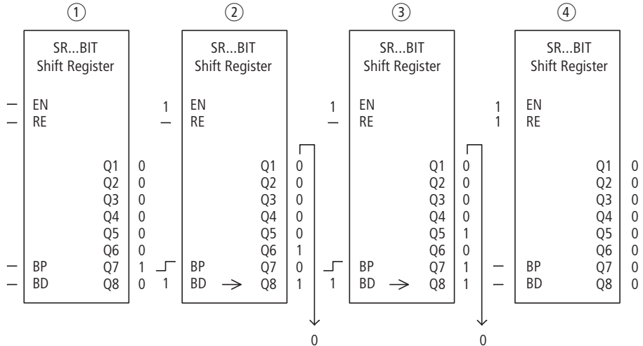
Figura 148: Registro di scorrimento SR...: operazione arretramento in modalità BIT
