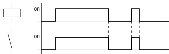
Figura 58: Diagramma di stato "funzione contattore"
