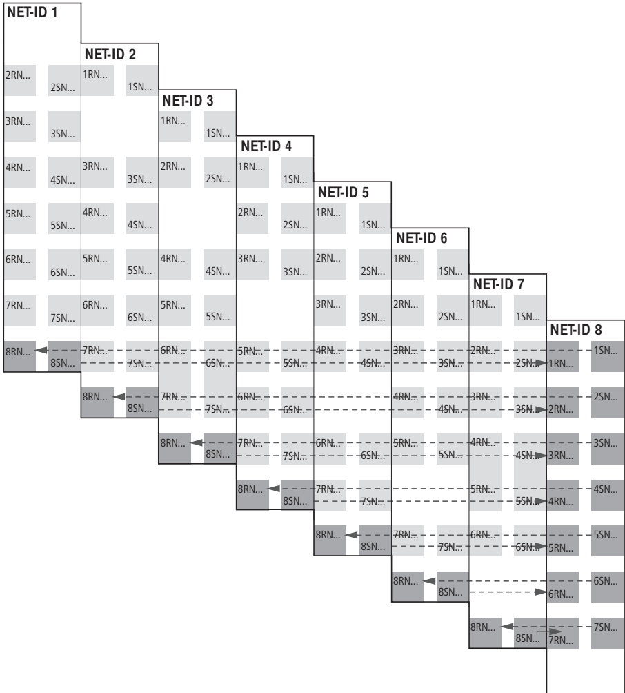
Figura 287: Combinazioni SN-RN dell'utente NET 8
