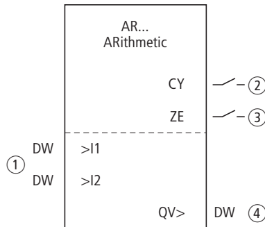
Figura 73: Modulo funzionale "aritmetico"
