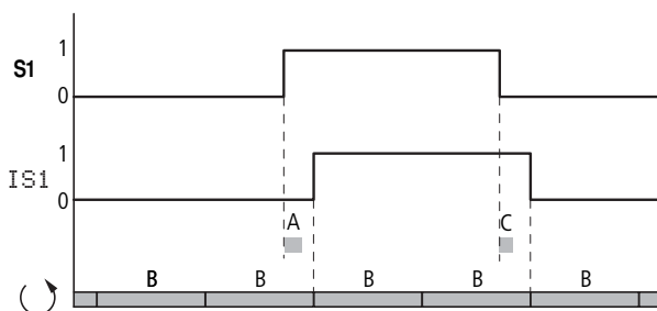
Figura 294: Comportamento alla commutazione con il FILTRO INGRESSI disattivato
