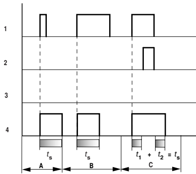
Figura 162: Diagramma di stato temporizzatore, a generazione di impulsi 1
