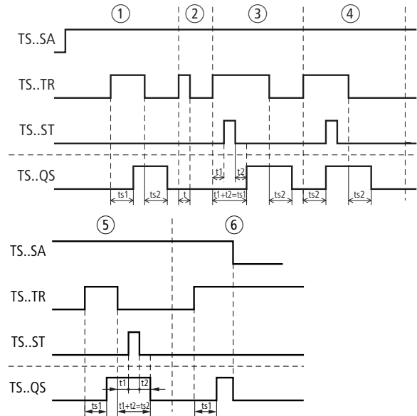
Figura 263: Diagramma d'azione "Temporizzatore, ritardato all'eccitazione e alla diseccitazione"
