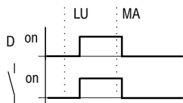
Figura 107: Diagramma di stato "Inserzione notturna"
