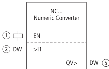
Figura 130: Modulo funzionale "Convertitore numerico"
