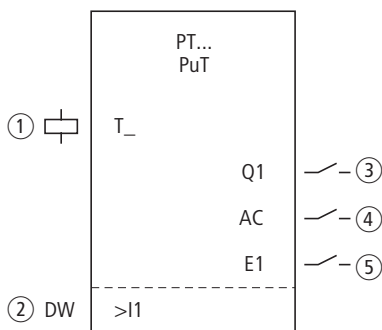
Figura 135: Modulo funzionale PUT
