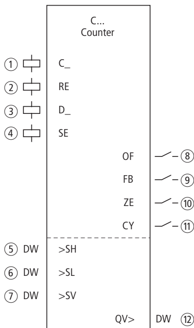
Figura 83: Modulo funzionale "Relè contatore"
