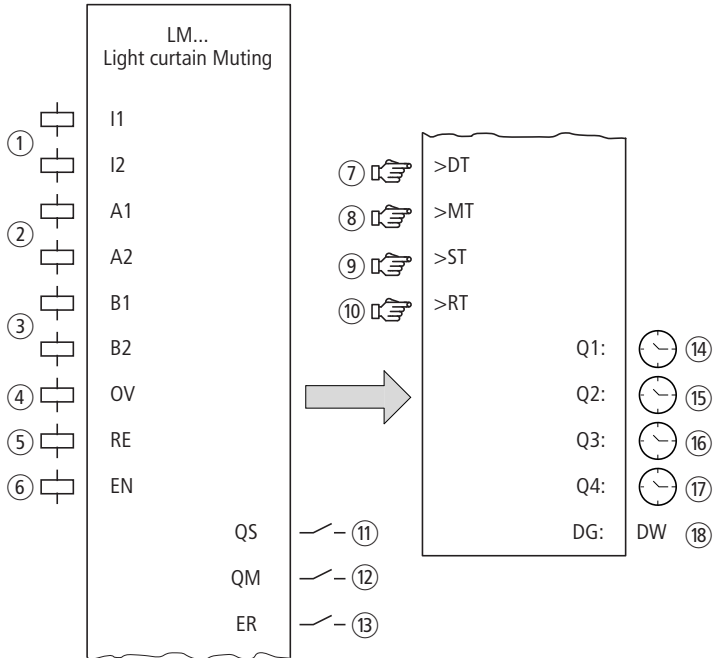
Figura 208: Modulo funzionale: "Muting griglia ottica"
