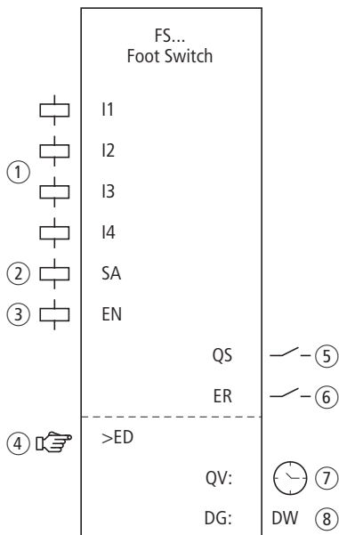
Figura 191: Modulo funzionale "Interruttore a pedale di sicurezza"
