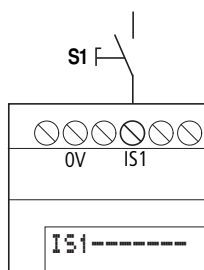
Figura 292: Ingresso easySafety configurato con interruttore
