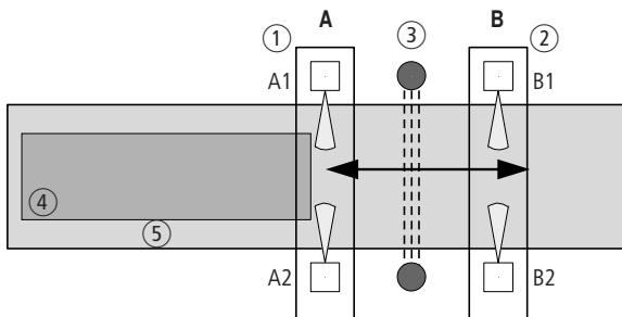
Figura 211: Muting griglia ottica: figura d'esempio, la direzione della freccia indica la possibile direzione del movimento del bene trasportato supportata dal procedimento di muting.
