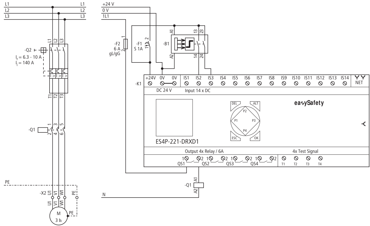
Figura 202: Esempio 1 "Griglia ottica" : schema elettrico
