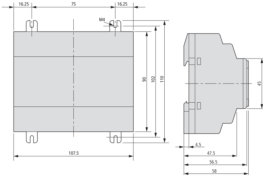
Figura 298: Dimensioni easySafety in mm (dati in pollici a tabella 37)
