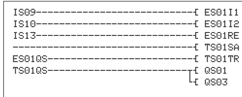
Figura 267: Esempio di arresto d'emergenza, categoria di arresto 1 in conformità alla norma EN IEC 60204-1: schema elettrico in easySafety
