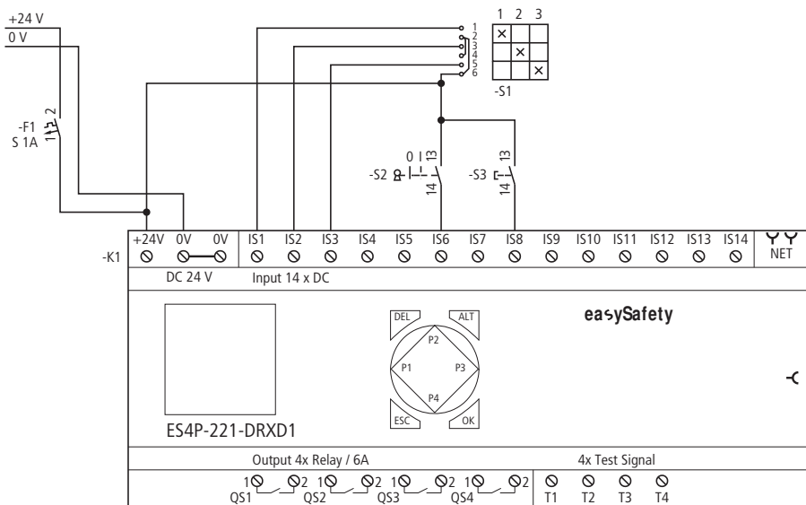
Figura 231: Esempio "Selettore modalità": schema elettrico
