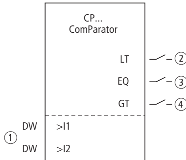
Figura 87: Modulo funzionale "Comparatore"
