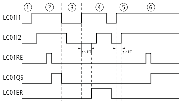
Figura 207: Esempio 2 "Griglia ottica": diagramma temporale
