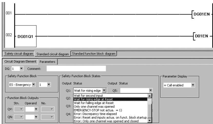
Figura 296: Assegnazione del modulo funzionale diagnostico e di sicurezza con easySoft-Safety
