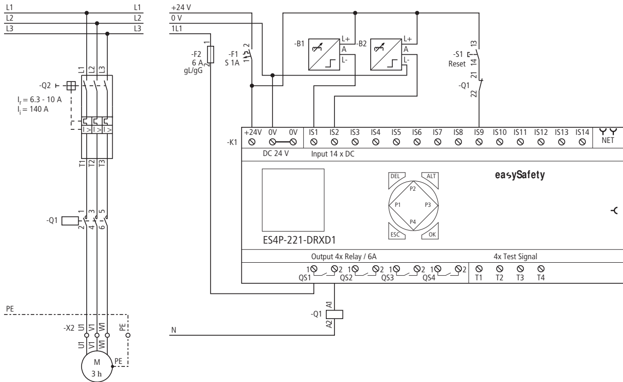
Figura 224: Esempio "Monitoraggio numero di giri massimo": schema elettrico
