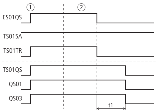
Figura 268: Esempio 2 Arresto d'emergenza: diagramma temporale
