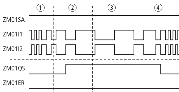
Figura 275: Esempio "Monitoraggio arresto": diagramma temporale
