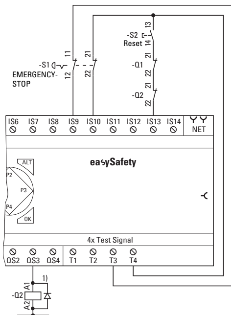
Figura 20: Esempio di impiego delle uscite a segnali di test in un collegamento dell'arresto d'emergenza a due canali. 1) Utilizzare diodi soppressori per apparecchi ES4P-221-DMX.. di versione 02 e 10
