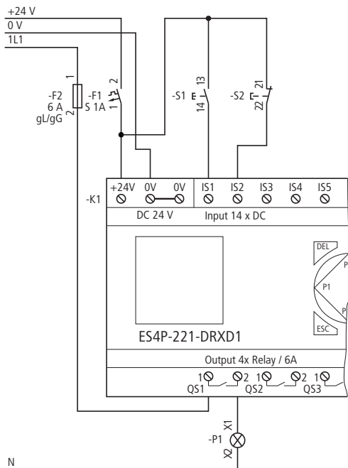
Figura 34: Comando lampade con un apparecchio easySafety
