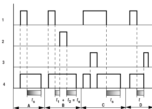
Figura 157: Diagramma di stato Temporizzatore ritardato alla diseccitazione (con/senza interventi casuali, con/senza riarmo)
