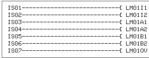
Figura 209: Schema elettrico easySafety con il modulo-funzionale Muting griglia ottica.
