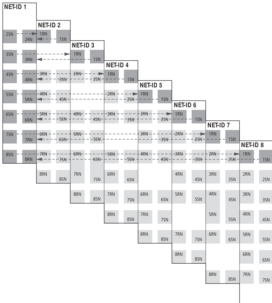
Figura 286: Combinazioni SN-RN dell'utente NET 1
