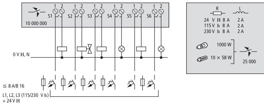
Figura 16: Uscite a relè EASY6...-RE..
