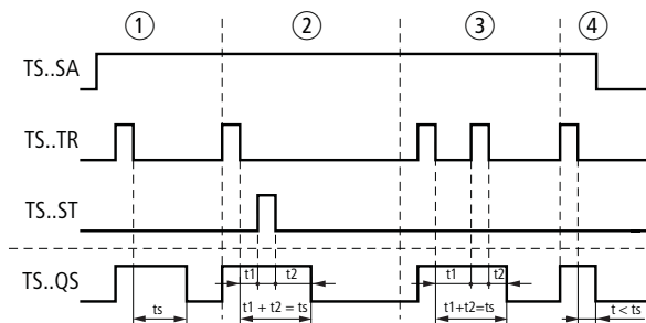
Figura 261: Diagramma d'azione "Temporizzatore ritardato alla diseccitazione"
