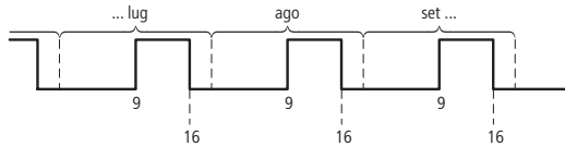
Figura 115: Selezionare determinati giorni in determinati mesi
