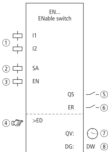
Figura 178: Modulo funzionale "Interruttore di approvazione"
