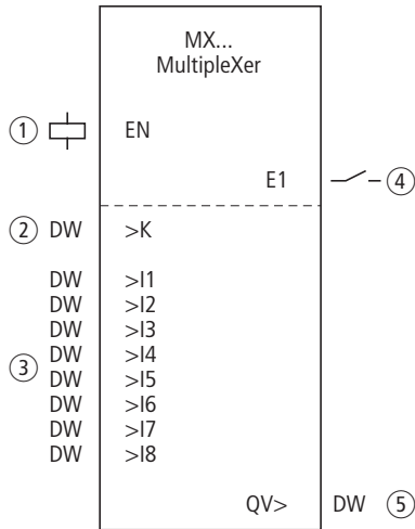
Figura 126: Modulo funzionale "Multiplexer dati"
