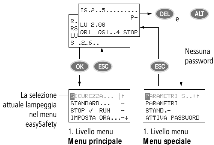
Figura 3: Commutazione tra menu principale e menu speciale
