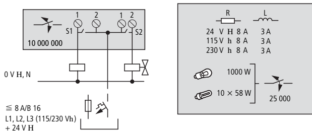
Figura 17: Uscite a relè EASY2...-RE..
