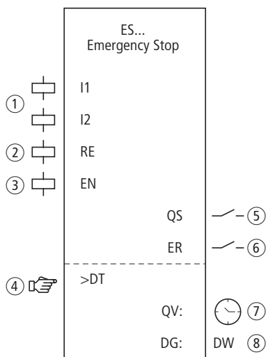
Figura 185: Modulo funzionale Arresto d'emergenza
