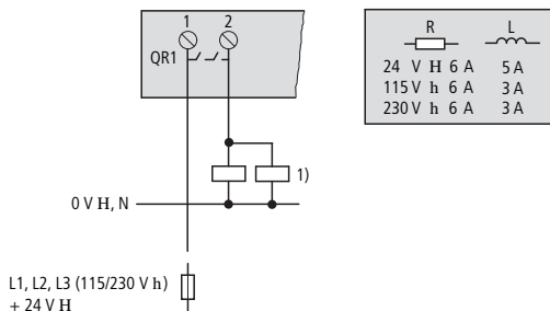
Figura 14: Uscita relè ridondante ES4P-221-DM...
