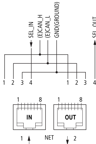
Figura 21: Connettori femmina RJ45
