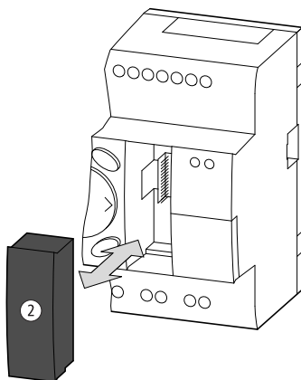
Figura 29: Inserimento e rimozione di una scheda di memoria ②
