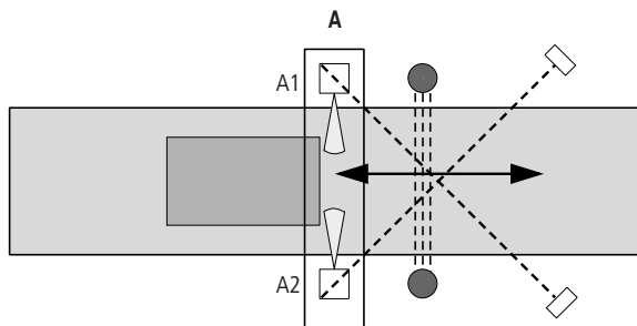
Figura 216: Muting griglia ottica: muting parallelo con 2 sensori muting
