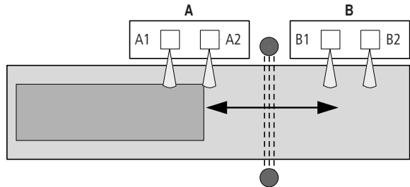
Figura 215: Muting griglia ottica: muting sequenziale con 4 sensori muting
