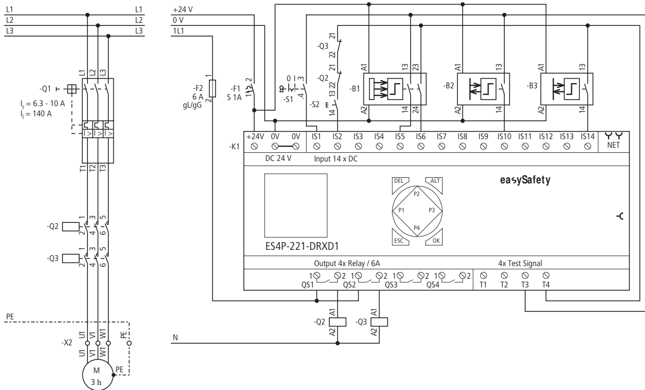
Figura 217: Esempio "Muting griglia ottica": schema elettrico
