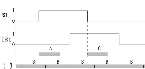
Figura 293: Tempi di ritardo nella valutazione di un segnale in ingresso e con FILTRO INGRESSI attivato
