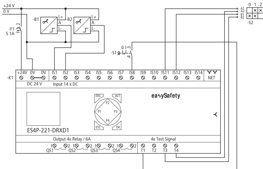
Figura 196: Esempio "Interruttore a pedale": schema elettrico
