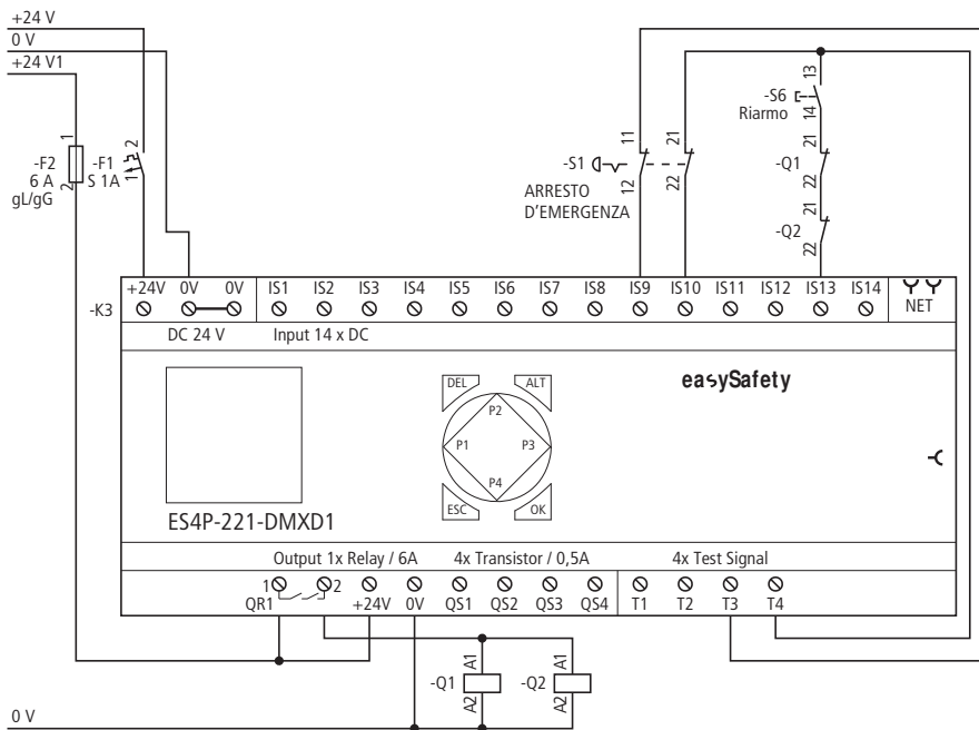
Figura 11: Esempio di applicazione dell'arresto d'emergenza, a due canali con apparecchio di base easySafety
