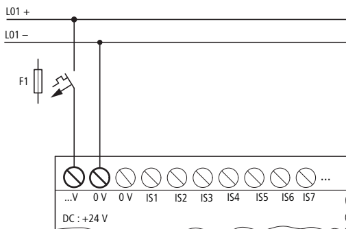
Figura 8: Tensione di alimentazione all'apparecchio base AC
