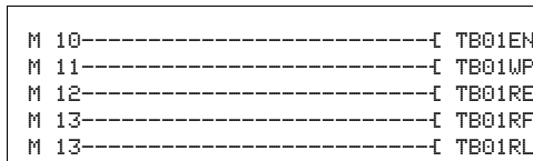
Figura 166: Cablaggio delle bobine del modulo
