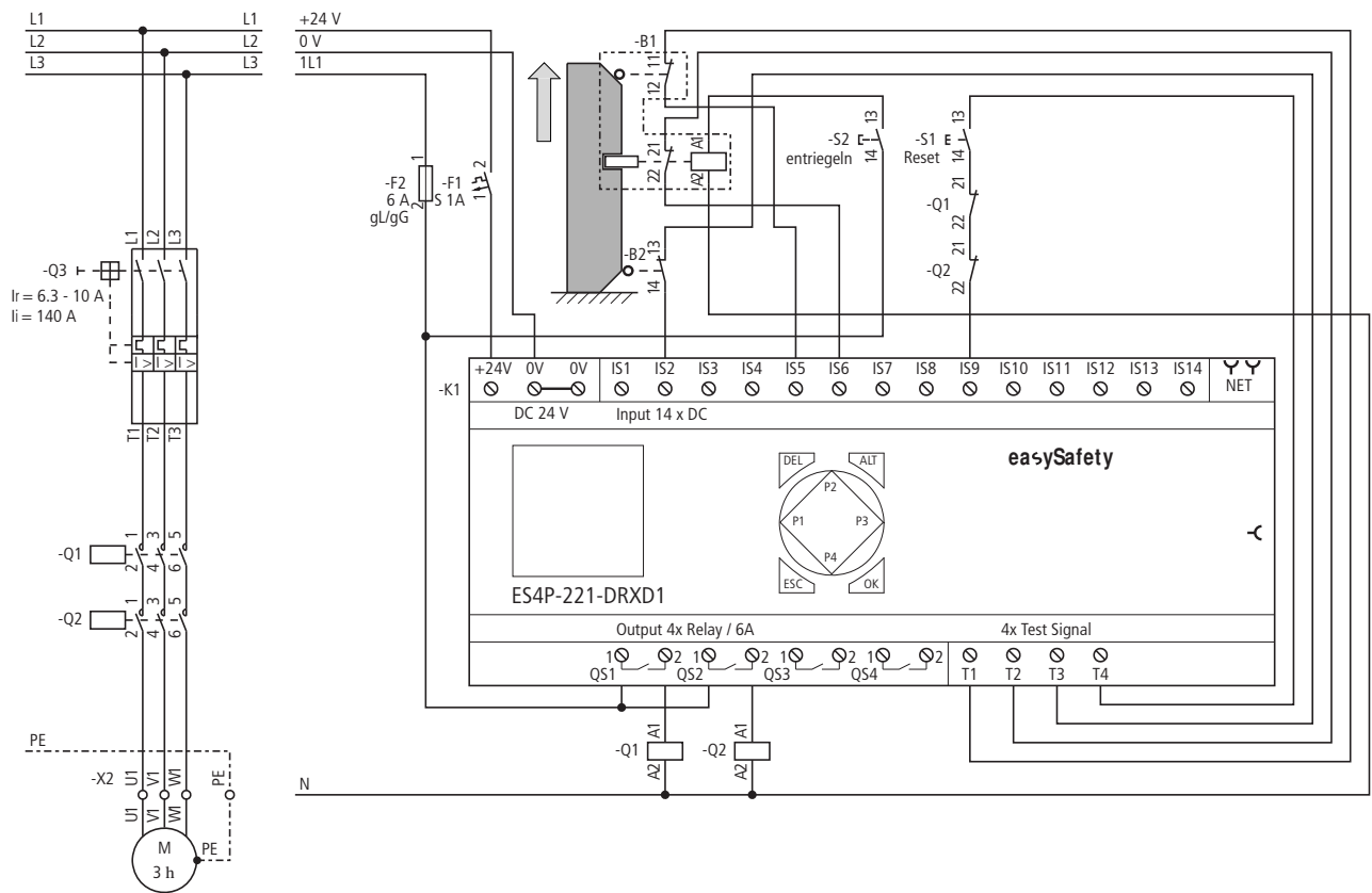
Figura 245: Esempio 2 "Porta di sicurezza": schema elettrico
