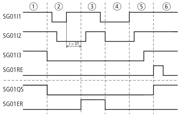
Figura 247: Esempio 2 "Porta di sicurezza": diagramma temporale
