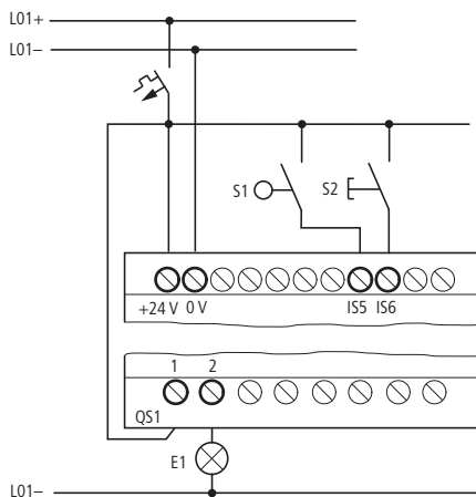
Figura 170: Cablaggio con easySafety ES4P...-DRX...
