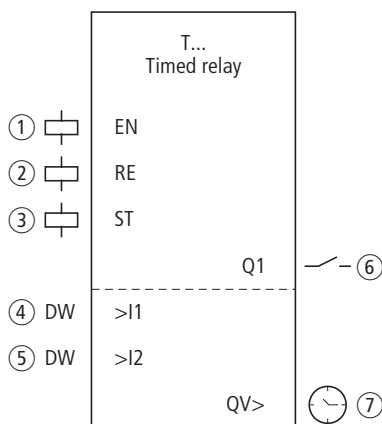
Figura 152: Modulo funzionale "Temporizzatore"
