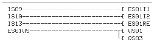
Figura 189: Esempio di arresto d'emergenza: schema elettrico in easySafety
