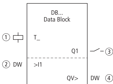
Figura 94: Modulo funzionale "Modulo dati"
