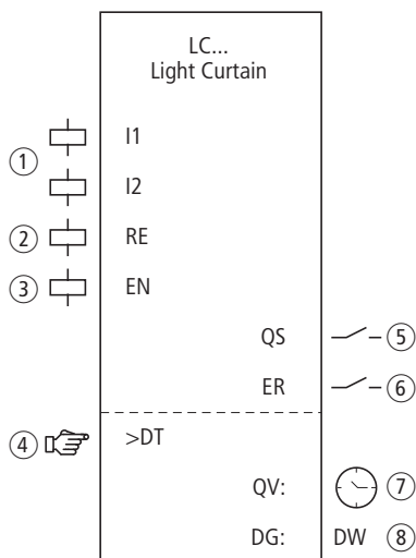
Figura 199: Modulo funzionale "Griglia ottica"
