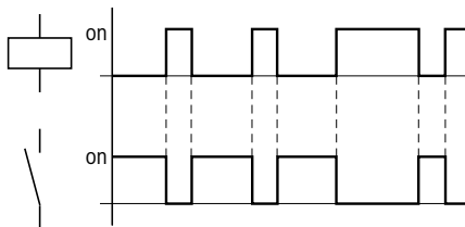
Figura 62: Diagramma di stato "funzione contattore inversa"
