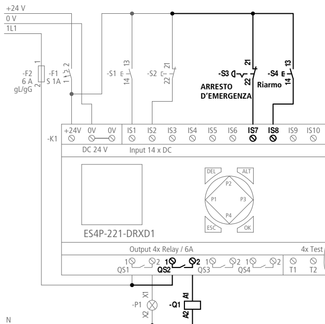
Figura 38: Circuito dell'arresto d'emergenza con un apparecchio easySafety (l'area di sicurezza è evidenziata nel grafico)
