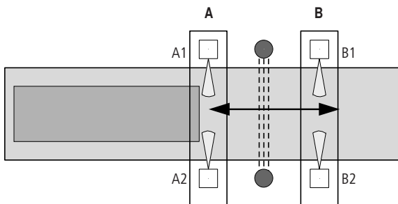
Figura 213: Muting griglia ottica: muting parallelo con 4 sensori muting
