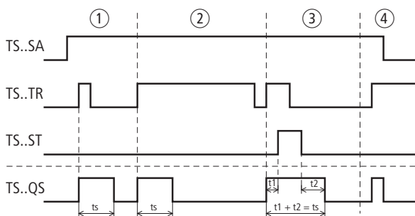
Figura 264: Diagramma di stato "Temporizzatore, a generazione di impulsi"
