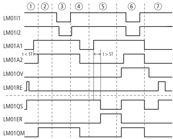
Figura 219: Esempio "Muting griglia ottica": diagramma temporale funzionamento indisturbato
