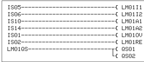
Figura 218: Esempio "Muting griglia ottica": schema elettrico in easySafety
