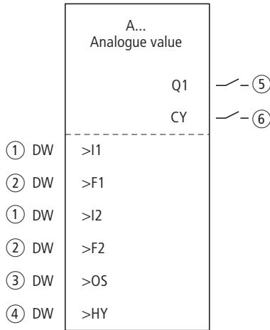
Figura 70: Modulo funzionale "Comparatore valore analogico"
