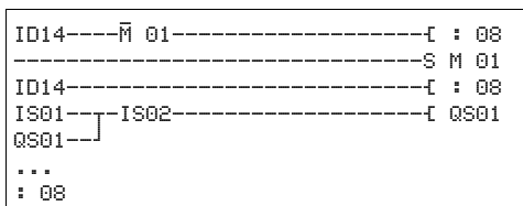
Figura 297: Schema elettrico standard per la verifica dell'espansione
