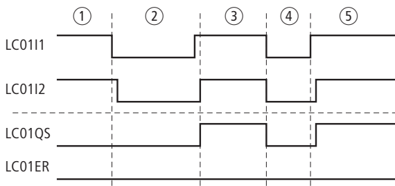
Figura 204: Esempio 1 "Griglia ottica": diagramma temporale
