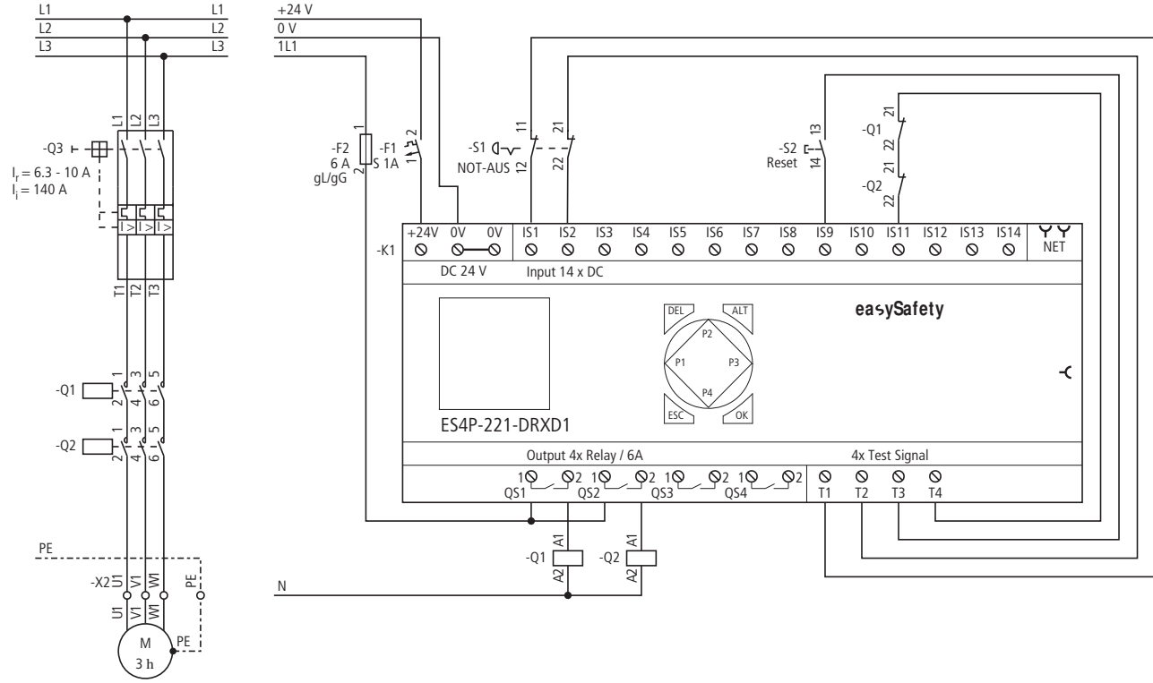
Figura 175: Esempio "Ritorno": schema elettrico
