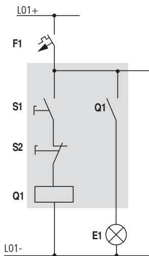
Figura 33: Comando di lampade tramite relè
