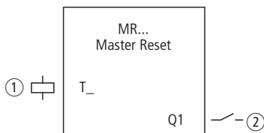
Figura 123: Modulo funzionale "Master reset"
