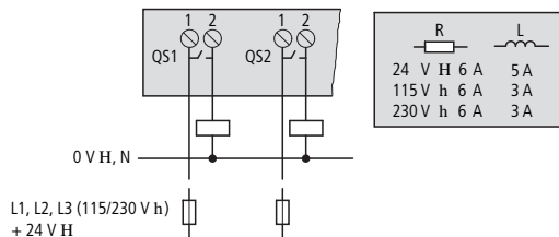
Figura 15: Uscite relè ES4P-221-DR...
