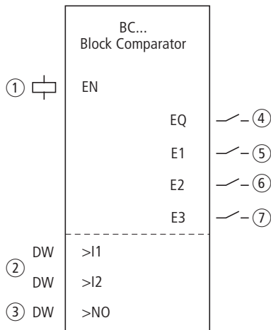
Figura 75: Modulo funzionale "Comparatore di blocchi dati"
