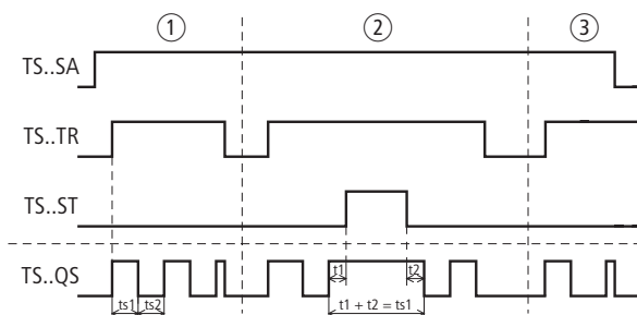
Figura 265: Diagramma d'azione "Temporizzatore, lampeggiamento sincrono e asincrono"
