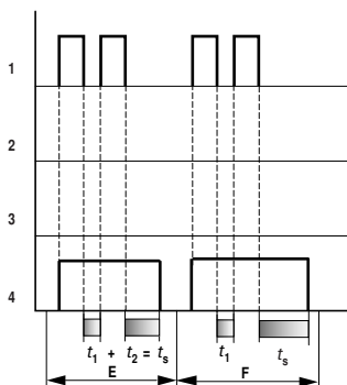
Figura 158: Diagramma di stato Temporizzatore ritardato alla diseccitazione (con/senza interventi casuali, con/senza riarmo)
