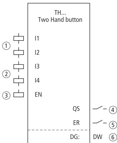
Figura 248: Modulo funzionale: "Tasto a due mani"
