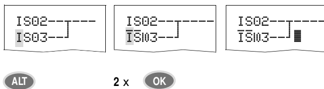
Figura 50: Modificare il contatto I503 da contatto NA a contatto NC
