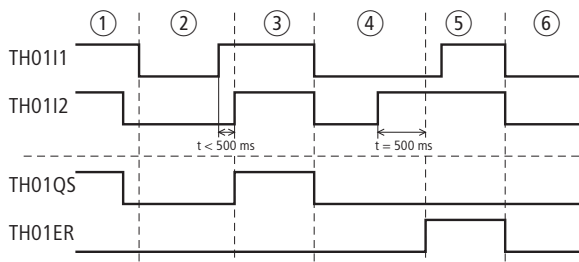
Figura 253: Esempio 1 "Tasto a due mani": diagramma temporale
