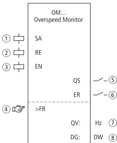
Figura 220: Modulo funzionale "Monitoraggio numero di giri massimo"
