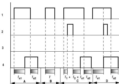
Figura 159: Diagramma di stato temporizzatore, ritardato all'eccitazione e alla diseccitazione 1
