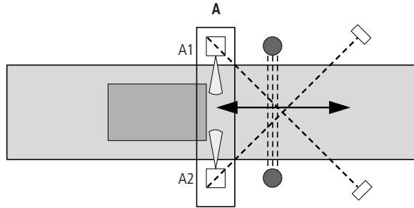
Figura 212: Muting griglia ottica: muting parallelo con 2 sensori muting
