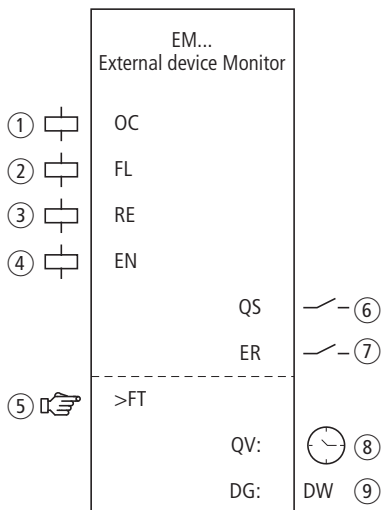
Figura 172: Modulo funzionale "Monitoraggio circuito di ritorno"
