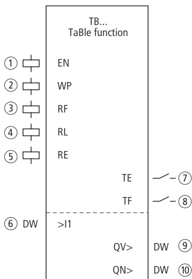
Figura 165: Modulo funzionale "Funzione tabelle"
