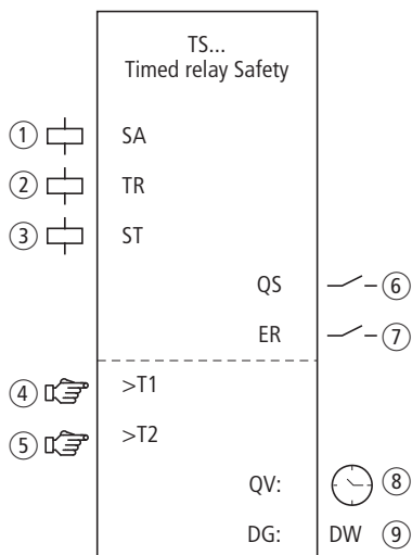
Figura 257: Modulo funzionale "Temporizzatore"
