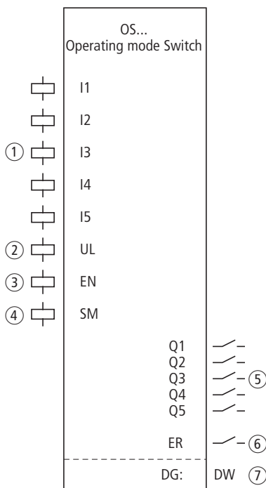
Figura 228: Modulo funzionale "Selettore delle modalità"
