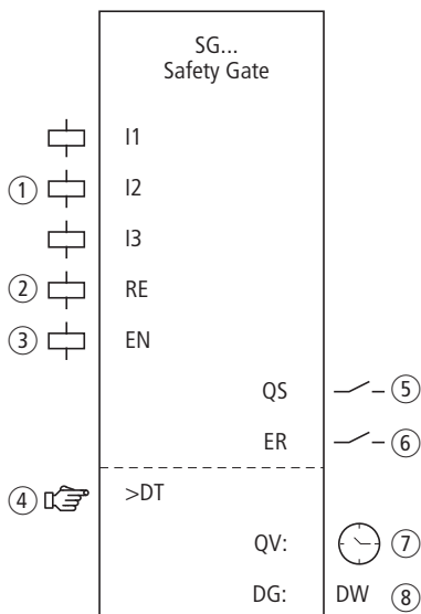
Figura 239: Modulo funzionale "porta di sicurezza"
