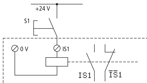
Figura 10: Collegare gli ingressi, in questo caso IS 1.
