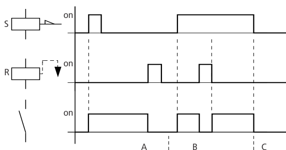
Figura 60: Diagramma di stato "Impostazione" e "Reset"
