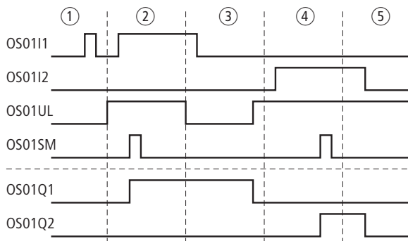
Figura 233: Esempio "selettore delle modalità": diagramma temporale
