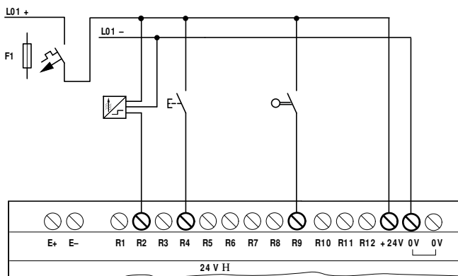
Figura 12: EASY6...-DC-.E (unità di espansione standard)
