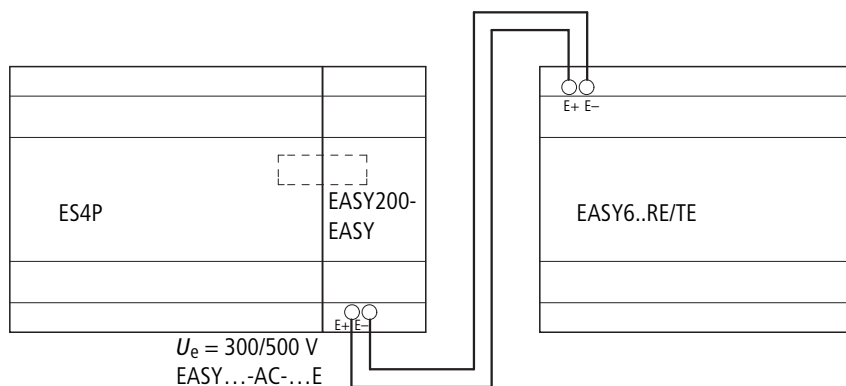
Figura 31: Collegare espansioni standard decentrate a easySafety
