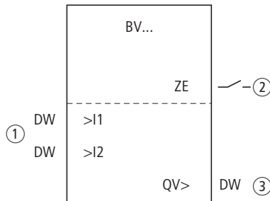
Figura 81: Modulo funzionale "Correlazione booleana"
