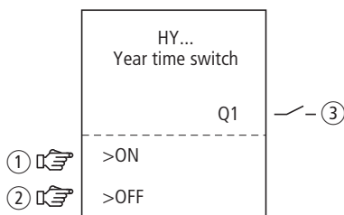
Figura 109: Modulo funzionale "temporizzatori annuali"
