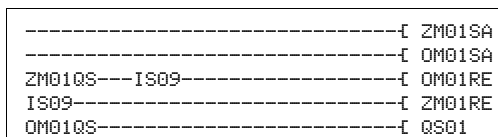
Figura 225: Esempio "Monitoraggio numero di giri massimo": schema elettrico in easySafety
