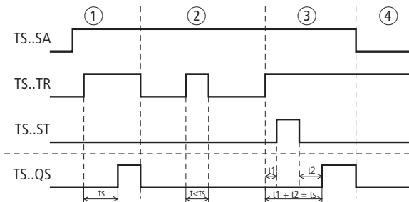
Figura 260: Diagramma d'azione "Temporizzatore ritardato all'eccitazione"
