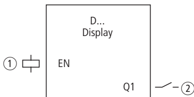
Figura 89: Modulo funzionale "Visualizzazione testo"
