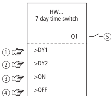
Figura 104: Modulo funzionale "Temporizzatore settimanale"
