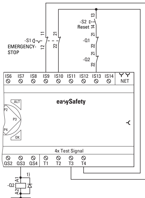
Figura 65: Utilizzo dei segnali di test 1) Utilizzare diodi soppressori per apparecchi ES4P-221-DMX.. di versione 02 e 10
