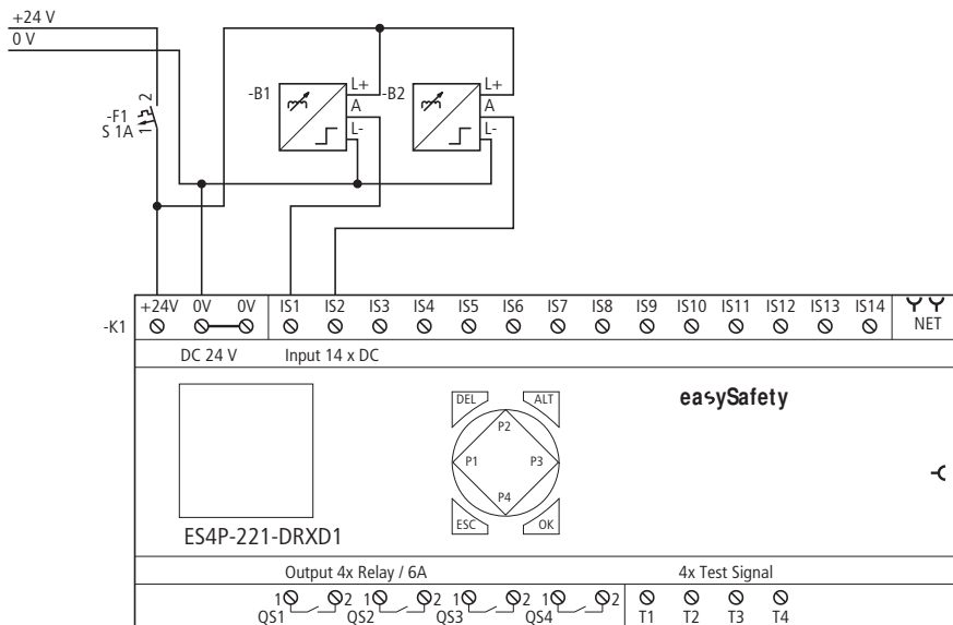
Figura 273: Esempio "Monitoraggio arresto": schema elettrico
