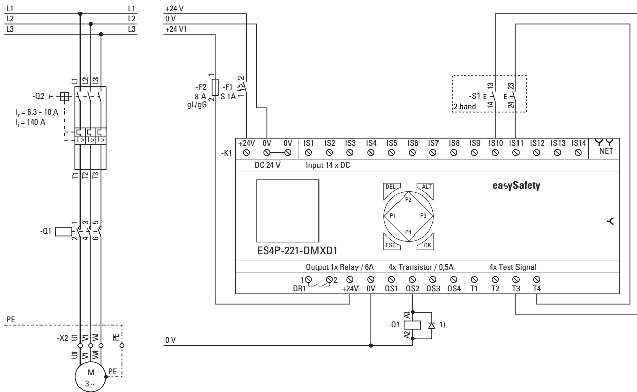
Figura 251: Esempio 1 "Tasto a due mani": schema elettrico
