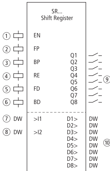
Figura 142: Modulo funzionale "Registro di scorrimento"
