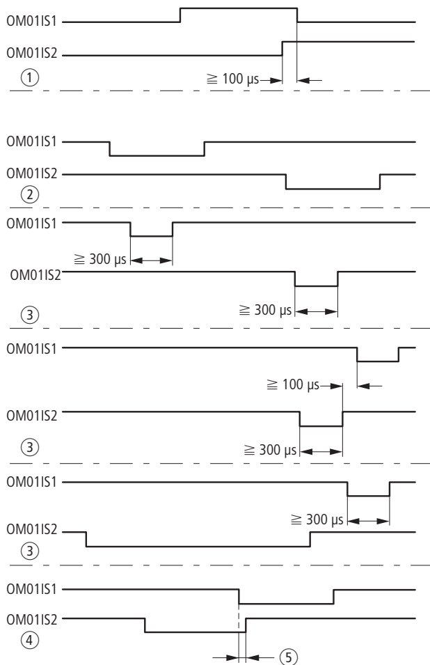
Figura 227: Andamento temporale dei segnali su IS1/IS2
