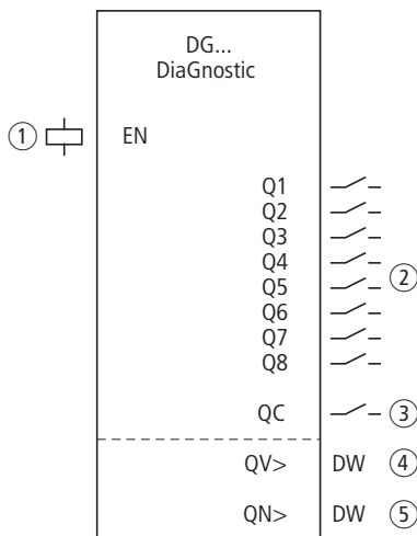
Figura 98: Modulo funzionale: "Diagnostico"
