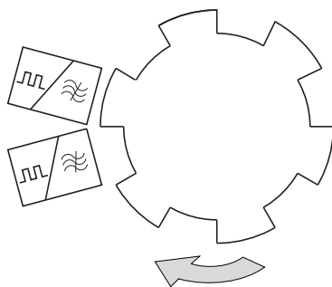
Figura 223: Monitoraggio del numero di giri massimo: rilevamento del numero di giri
