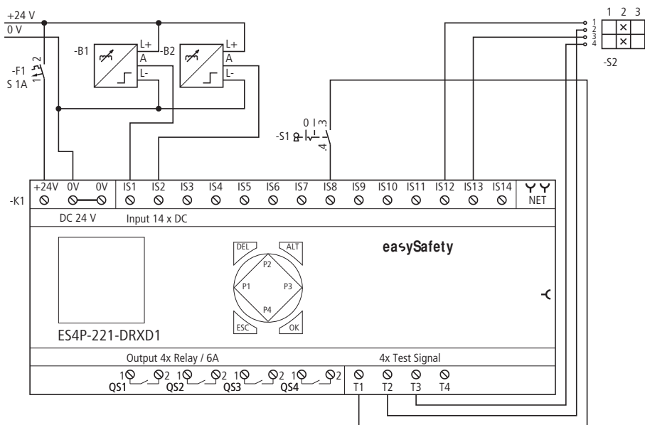
Figura 182: Esempio "Interruttore di approvazione" : schema elettrico
