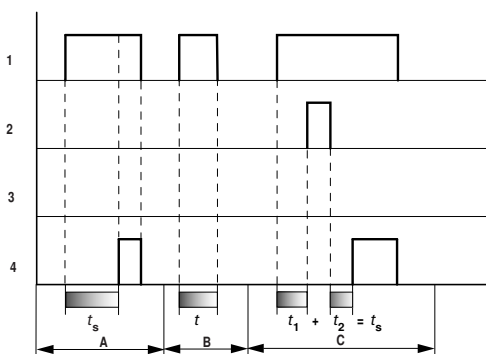
Figura 155: Diagramma di stato temporizzatore ritardato all'eccitazione (con/senza interventi casuali)
