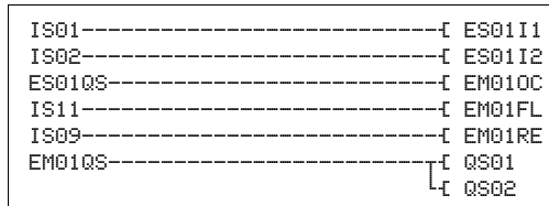
Figura 176: Esempio "Ritorno": schema elettrico in easySafety
