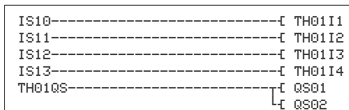
Figura 255: Esempio 2 "Tasto a due mani": schema elettrico in easySafety
