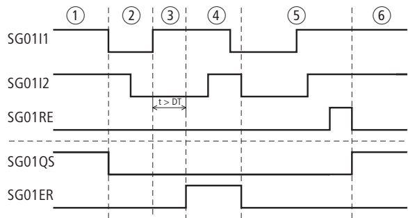
Figura 244: Esempio 1 "Porta di sicurezza": diagramma temporale
