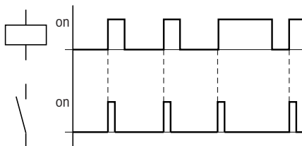
Figura 63: Diagramma di stato "impulso di ciclo" con fronte positivo
