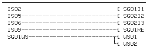
Figura 246: Esempio 2 "Porta di sicurezza": schema elettrico in easySafety
