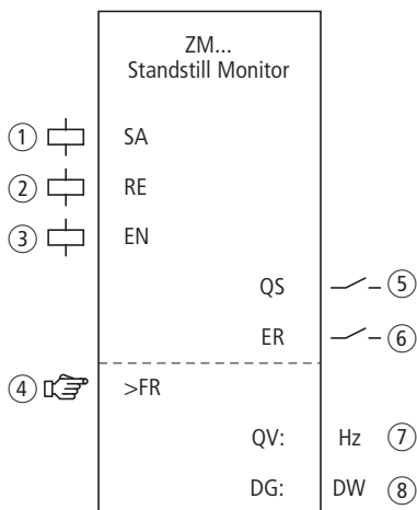
Figura 269: Modulo funzionale "Monitoraggio arresto"
