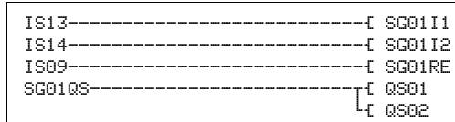
Figura 243: Esempio 1 "Porta di sicurezza": schema elettrico in easySafety
