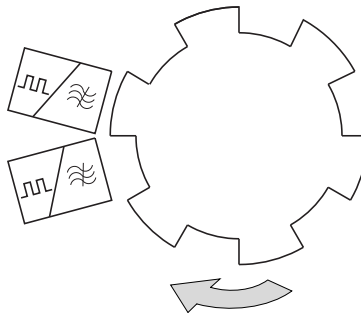
Figura 272: Monitoraggio arresto: misurazione regime
