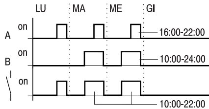
Figura 108: Diagramma di stato sovrapposizioni
