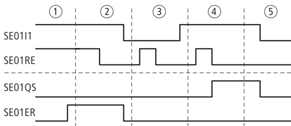
Figura 238: Esempio "Elemento di avvio": diagramma temporale
