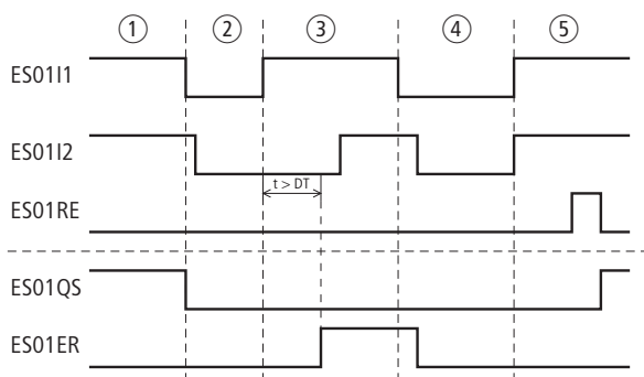
Figura 190: Esempio Arresto d'emergenza: diagramma temporale
