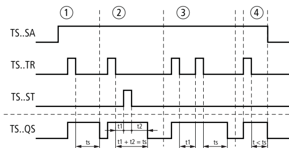
Figura 262: Diagramma d'azione "Temporizzatore ritardato alla diseccitazione" (con/senza ripetizione scatto)
