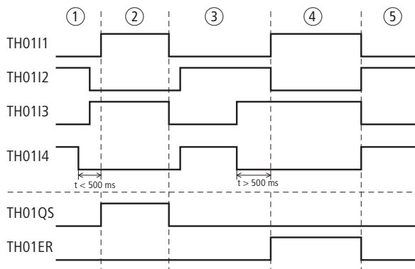
Figura 256: Esempio 2 "Tasto a due mani": diagramma temporale
