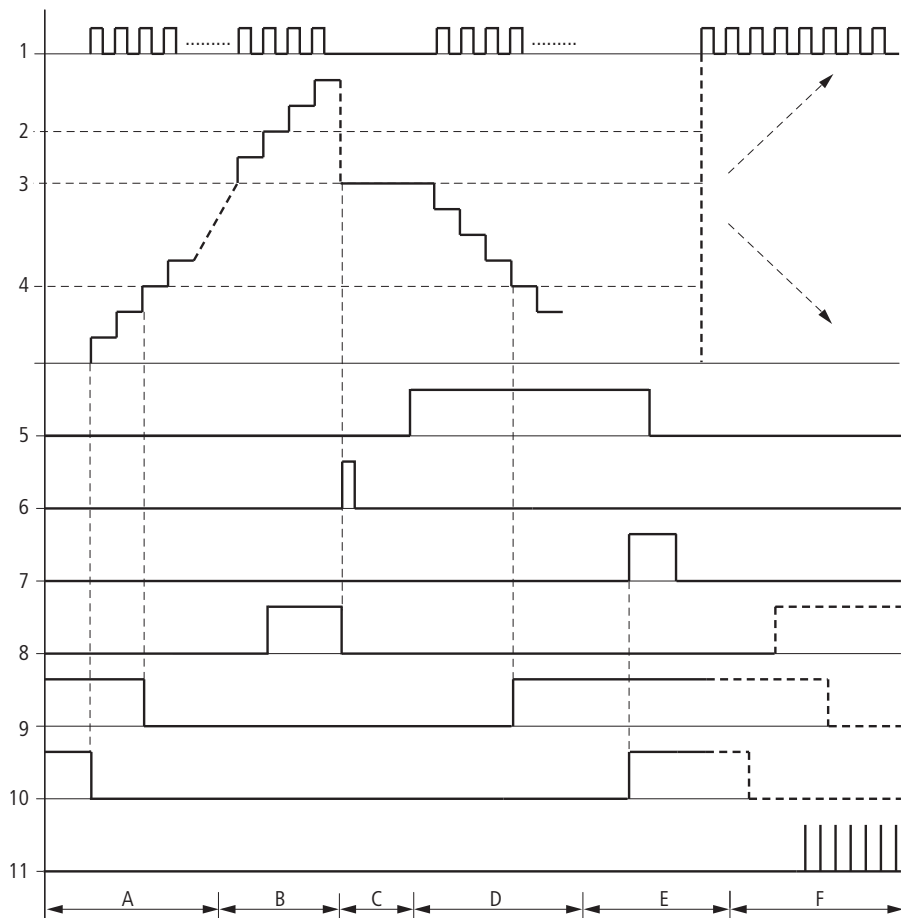
Figura 86: Diagramma di stato Relè di conteggio
