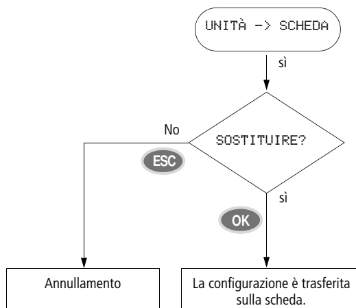
Figura 47: Salvare la configurazione sulla scheda.
