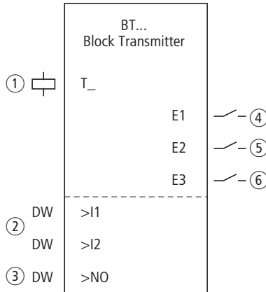
Figura 78: Modulo funzionale "Trasmissione blocco dati"
