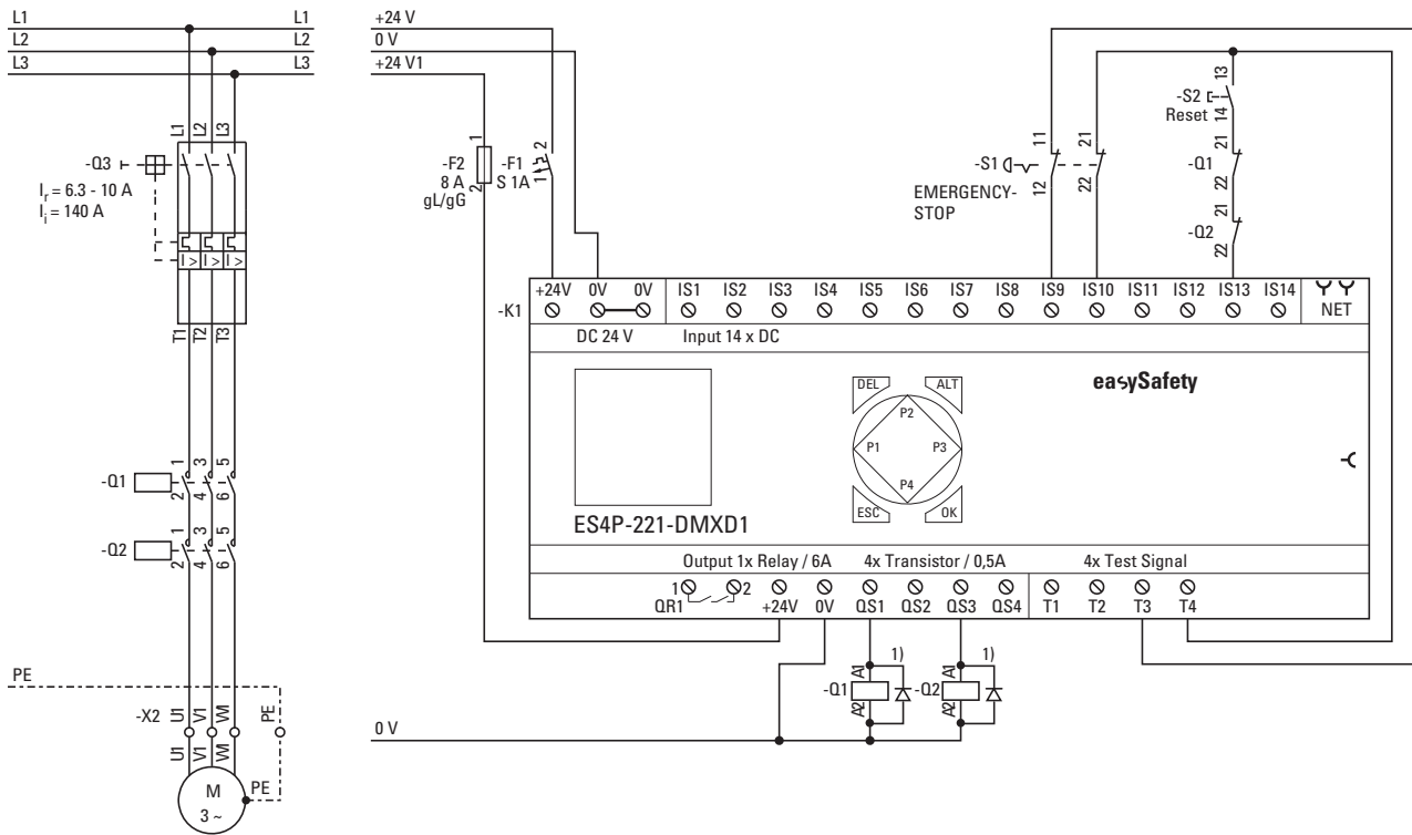
Figura 188: Esempio arresto d'emergenza: schema elettrico 1) Utilizzare diodi soppressori per apparecchi ES4P-221-DMX.. di versione 02 e 10
