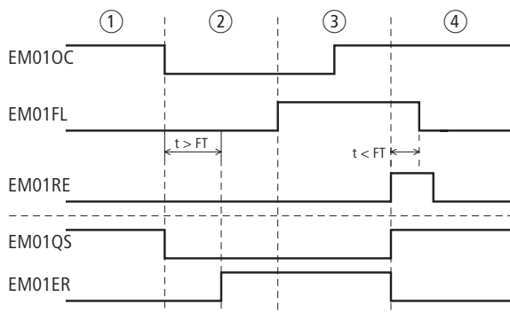
Figura 177: Esempio di ritorno: diagramma temporale
