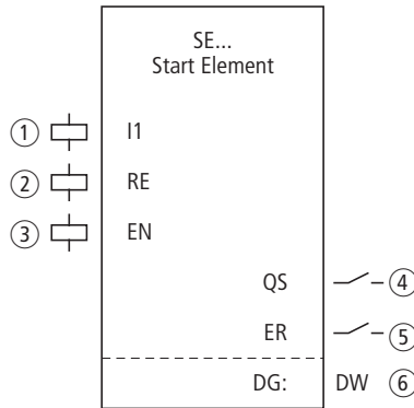
Figura 234: Modulo funzionale "Elemento di avvio"
