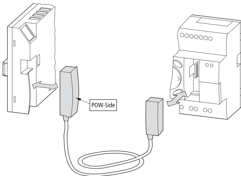
Figura 27: Inserire il connettore di collegamento: a sinistra MFD-CP..., a destra easySafety
