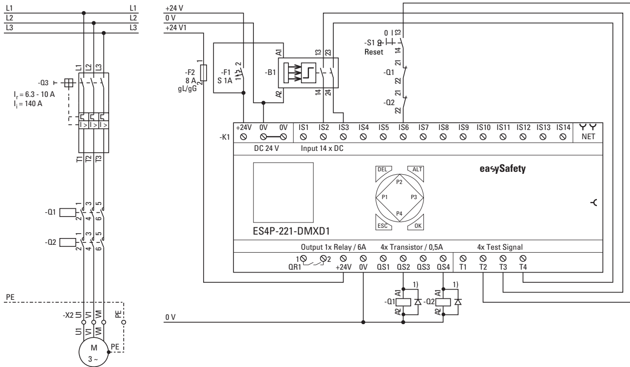
Figura 205: Esempio 2 "Griglia ottica" : schema elettrico 1) Utilizzare diodi soppressori per apparecchi ES4P-221-DMX.. di versione 02 e 10
