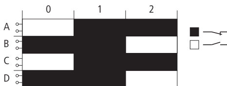
Figura 195: Contatto dell'interruttore a pedale a 4 canali con tre livelli 0, 1, 2 e quattro contatti A, B, C e D
