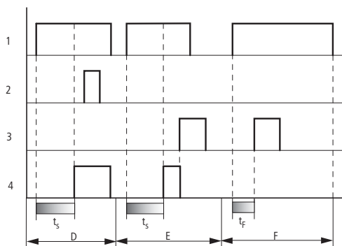
Figura 156: Diagramma di stato temporizzatore ritardato all'eccitazione (con/senza interventi casuali)
