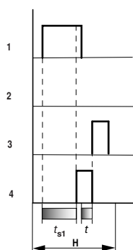
Figura 161: Diagramma di stato temporizzatore, ritardato all'eccitazione e alla diseccitazione 3
