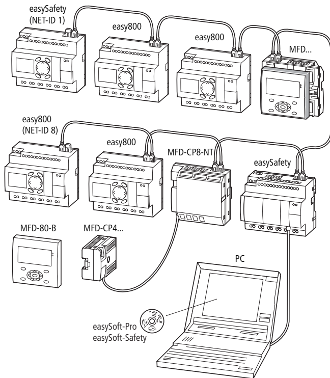
Figura 276: Gestione mista degli utenti NET
