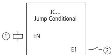
Figura 120: Modulo funzionale "Salto condizionato"
