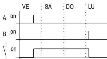
Figura 106: Diagramma di stato "Fine settimana"
