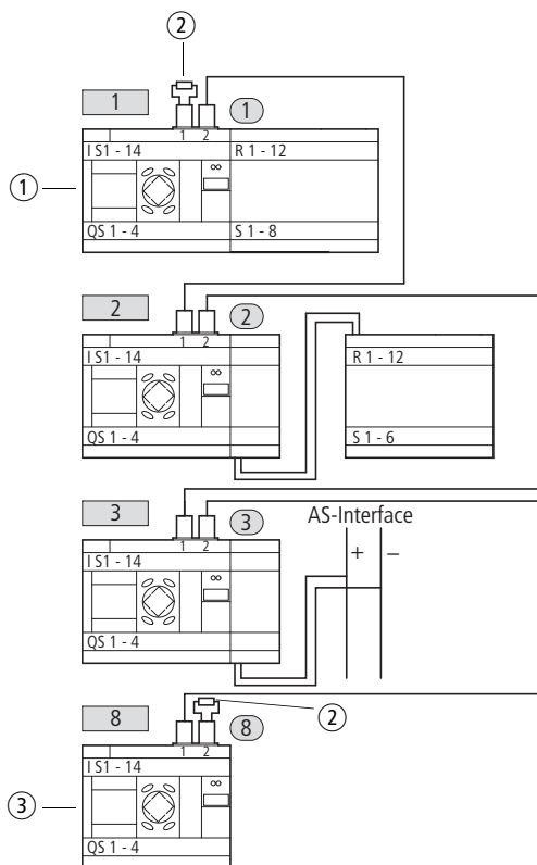
Figura 23: Resistenze di terminazione bus
