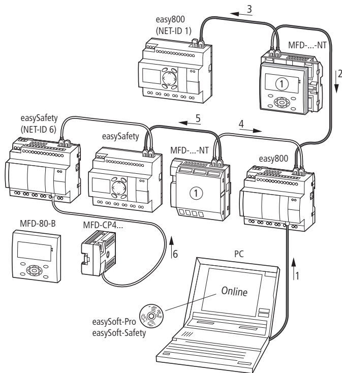
Figura 277: Possibilità di accesso in modalità terminale
