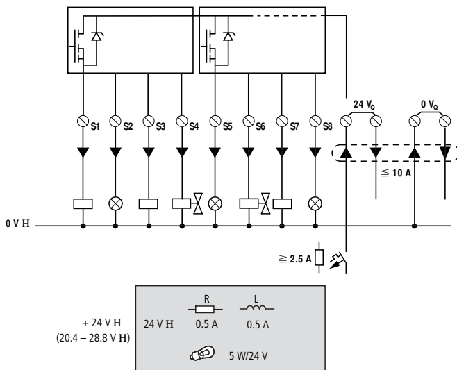
Figura 19: Uscite a transistor EASY6...-DC-TE
