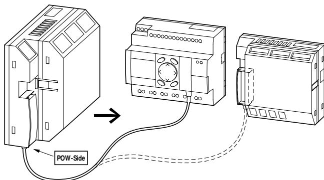
Figura 28: Connessione punto-punto dell'interfaccia seriale
