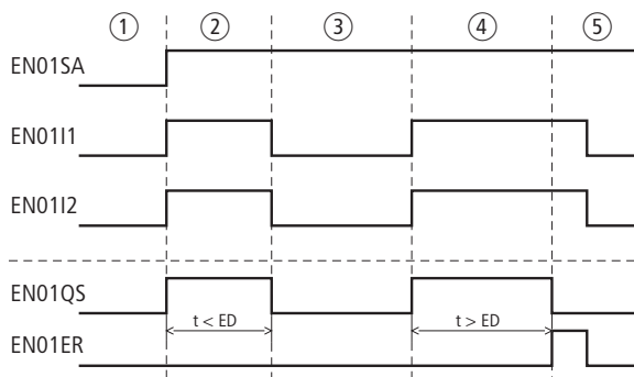
Figura 184: Esempio "Interruttore di approvazione":
