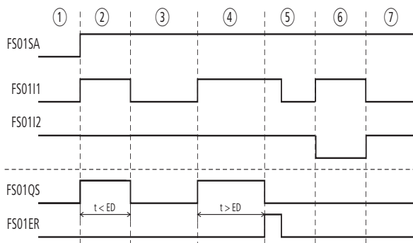
Figura 198: Esempio "Interruttore a pedale": diagramma temporale
