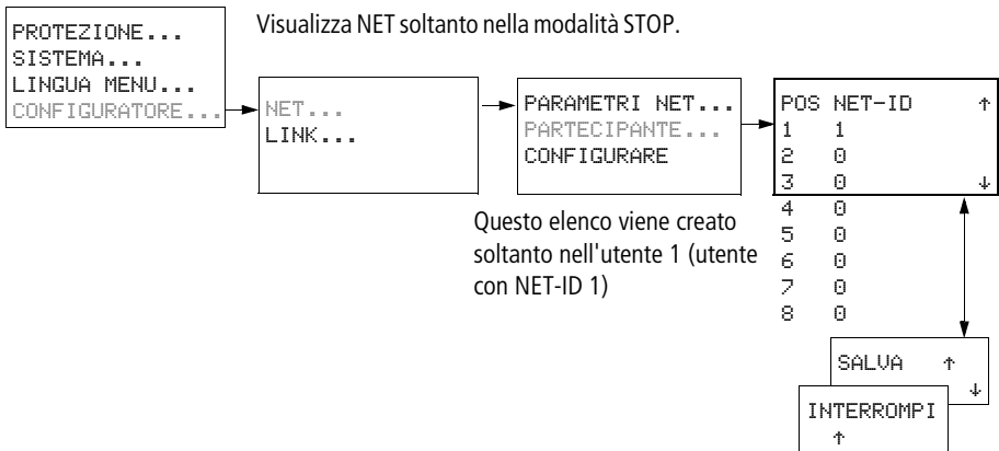
Figura 280: Menu PARTECIPANTE
