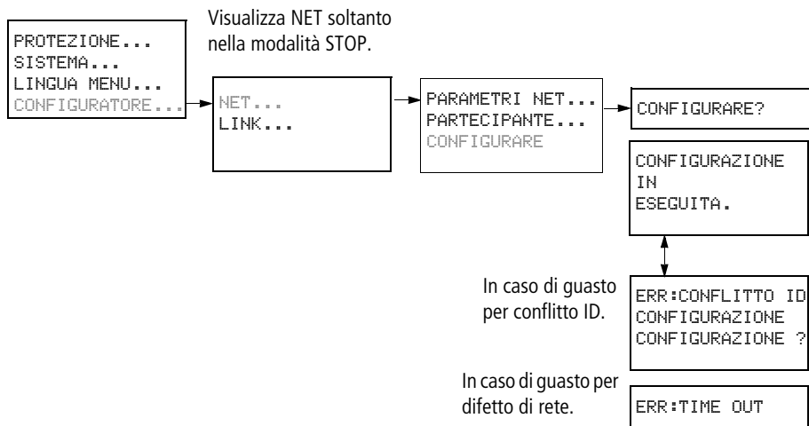
Figura 281: Menu CONFIGURARE
