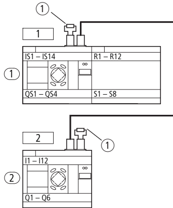
Figura 278: Esempio di topologia con due utenti NET
