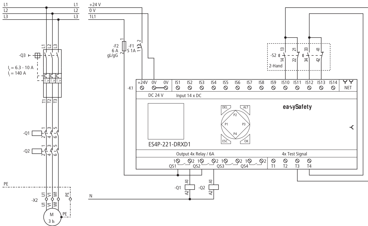
Figura 254: Esempio 2 "Tasto a due mani": schema elettrico
