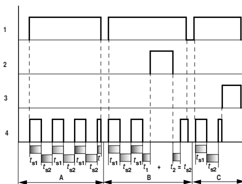
Figura 164: Diagramma di stato "Temporizzatore", lampeggiante in modo sincrono e asincrono
