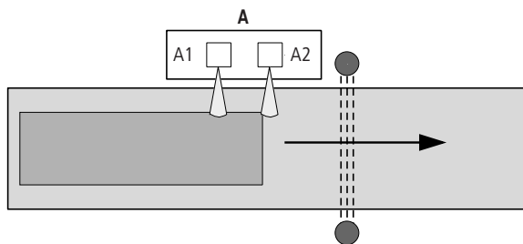
Figura 214: Muting griglia ottica: muting sequenziale con 2 sensori muting
