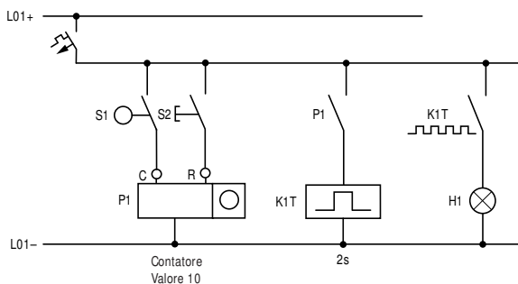
Figura 169: Cablaggio fisso con relè
