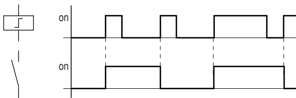
Figura 59: Diagramma d'azione "Relè passo-passo"
