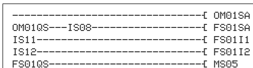
Figura 197: Esempio "Interruttore a pedale": schema elettrico in easySafety
