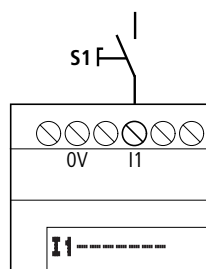
Abbildung 91: easy-Eingang mit Schalter belegt
