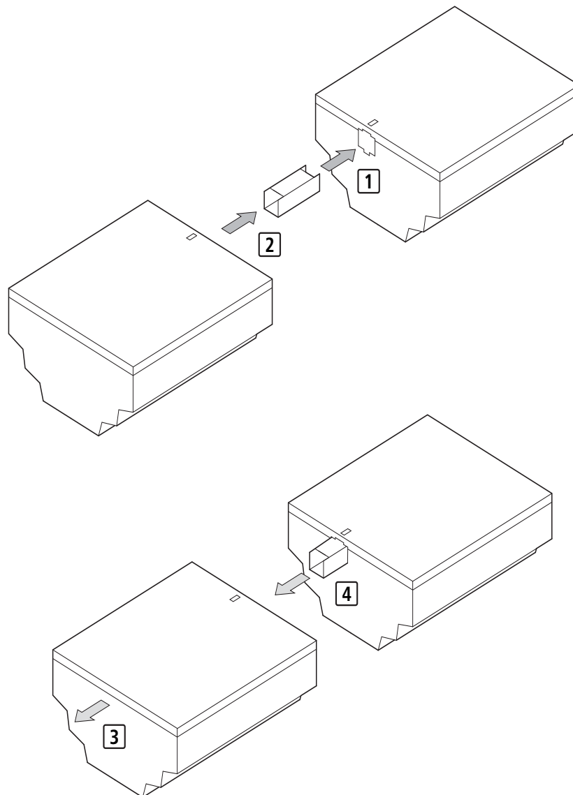
Abbildung 6: Erweiterungen anschließen
