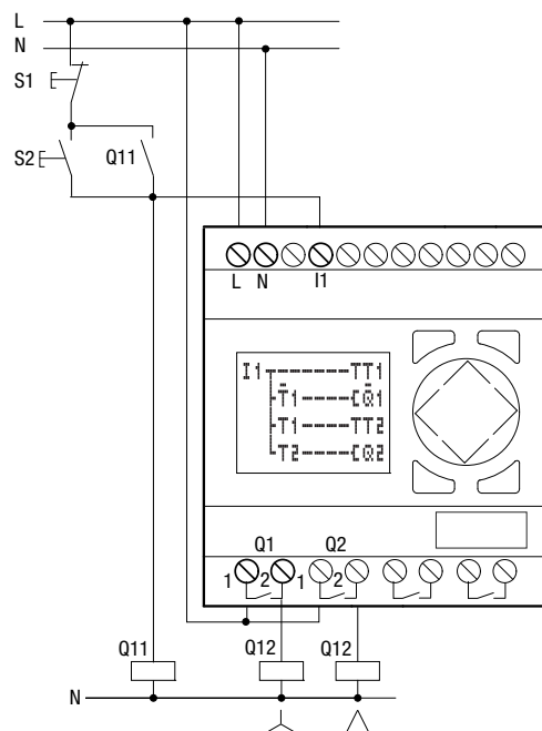
Abbildung 84: Stern-Dreieckschaltung mit easy
