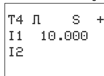
Parametereinstellungen des Zeitrelais T4
