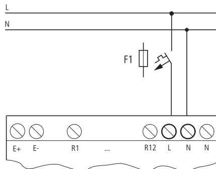
Abbildung 8: Versorgungsspannung an Erweiterungsgesicht AC
