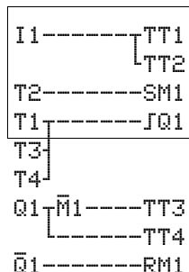
Abbildung 90: easy-Schaltplan Treppenhaus
