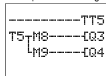
Schaltplandarstellung
