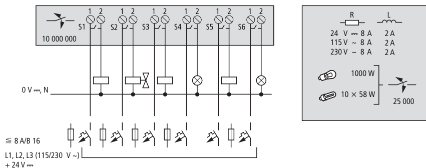
Abbildung 30:Relais-Ausgänge EASY618...-RE
