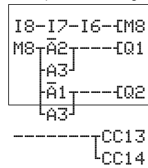
Schaltplandarstellung
