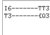
Schaltplandarstellung
