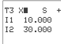
Parametereinstellungen des Zeitrelais T3
