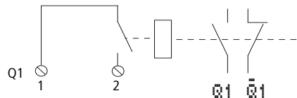
Abbildung 27: Ausgang Q
