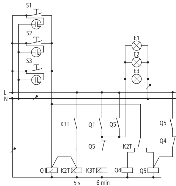
Abbildung 88: Konventionelle Treppenhausbeleuchtung
