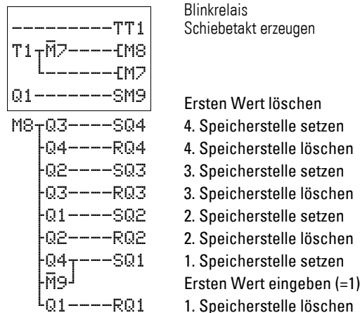
Abbildung 87: easy-Schaltplan Lauflicht
