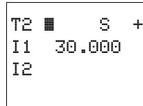
Parametereinstellungen des Zeitrelais T2
