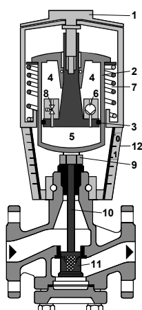
Клапан открыт
