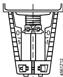
Цилиндр с полностью задвинутым коннектором штока клапана
