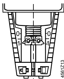
Цилиндр с полностью выдвинутым коннектором штока клапана
