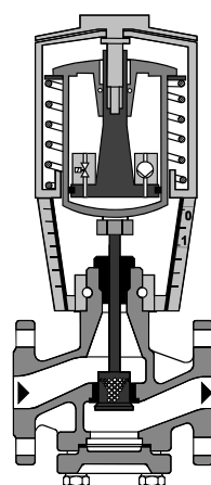
Клапан закрыт
