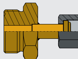
Адаптер, модель GCA Со страницы 11
