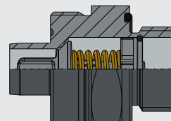
Клапан, модель GCV-20 Со страницы 2
