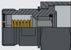
Клапан-соединитель, модель GCC-20 Со страницы 8
