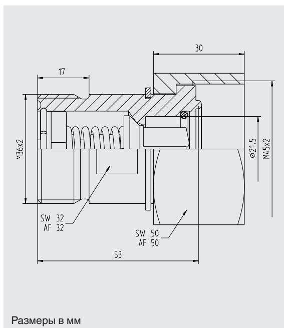
Адаптер, модель GCA Со страницы 11
