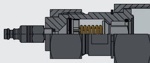
Подключение к аналитическим приборам, модель GCG-20 смотри страницу 10
