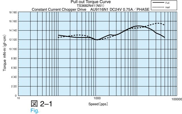
ドライバ Driver AU9116N1
