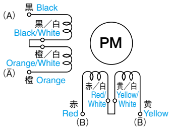
TYPE 3 バイポーラ(シリーズ結線) BIPOLAR SERIES (Series connection)
