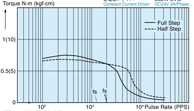
TS3653N3E8,N13E8
