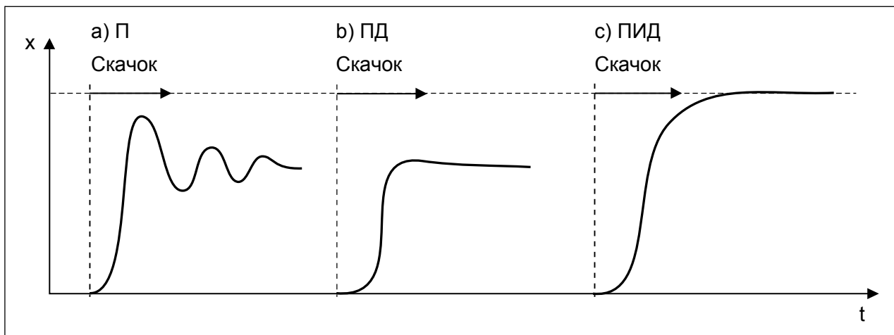
Рисунок 55: Настройка ПИД-регулятора эмпирическим методом
