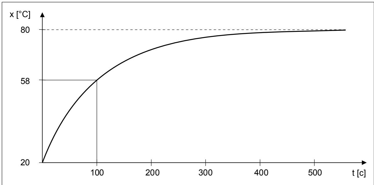
Рисунок 26: Примерный график переходной характеристики объекта 1-го порядка
