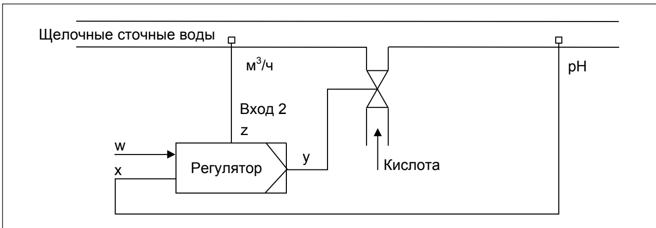
Рисунок 79: Нейтрализационная установка
