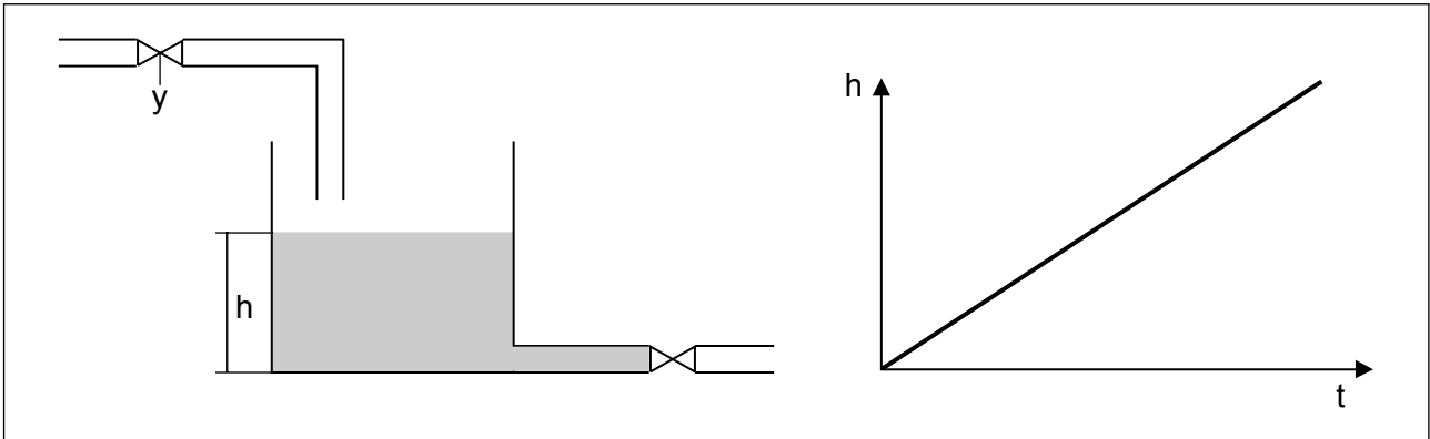
Рисунок 21: Объект с регулированием уровня жидкости
