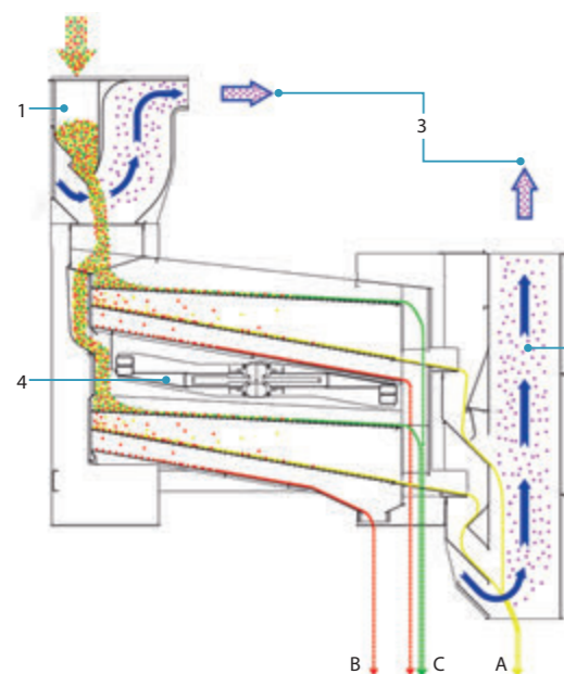
Схема SMA 206-6 Производительность до 400 т/ч
