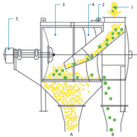
Схема скальператора МКЗМ Производительность до 500 т/ч
