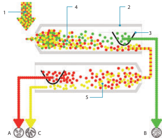
Схема Триера UN Производительность до 48 т/ч
