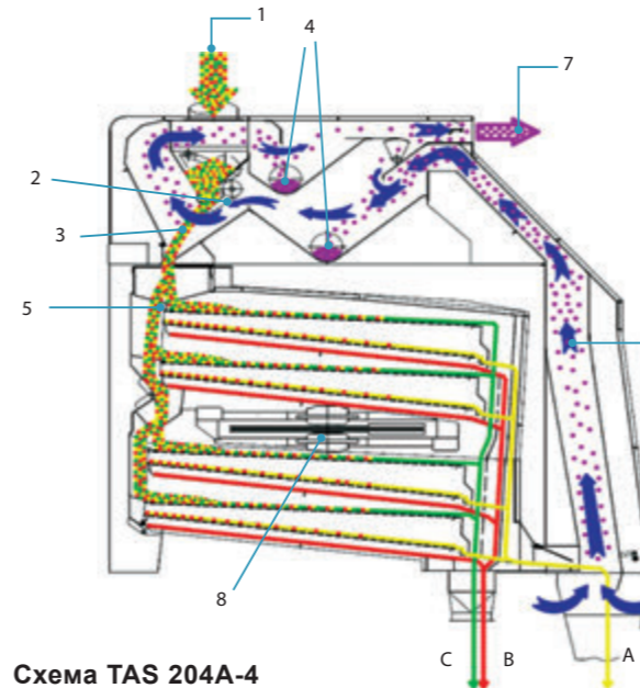
Схема TAS 204A-4 Производительность 160 т/ч
