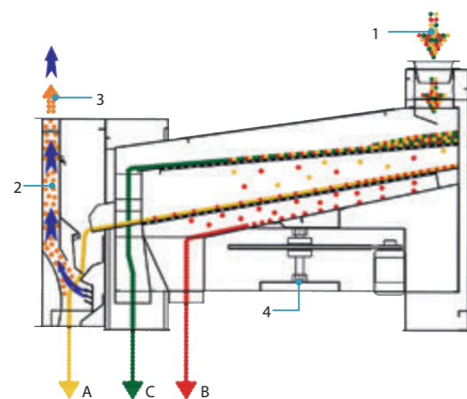
Схема SMA 05/10/20 Производительность 25-95 т/ч
