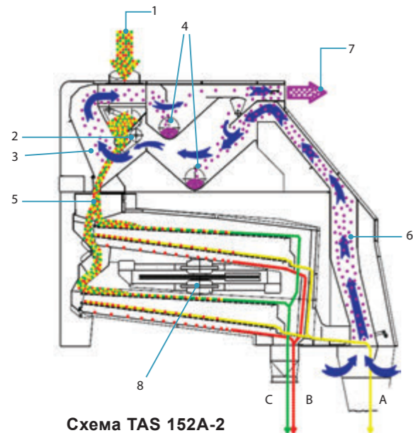
Схема TAS 152A-2 Производительность 60 т/ч
