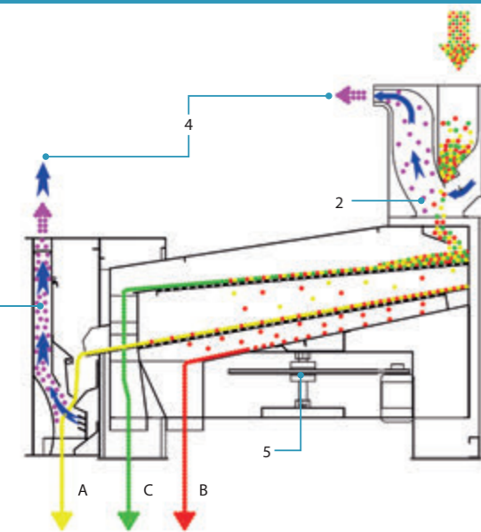
Схема GrainPlus с аспирацией на входе и выходе Производительность 25-95 т/ч
