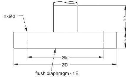
Flange (DIN 2501)
