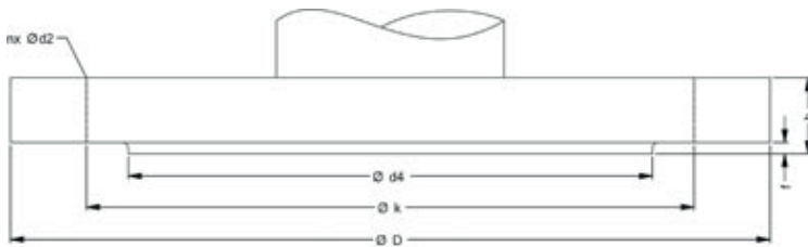
flange (DIN 2501)
