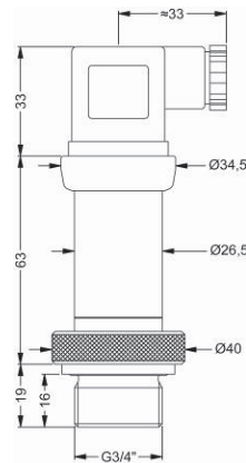
G3/4" DIN 3852
