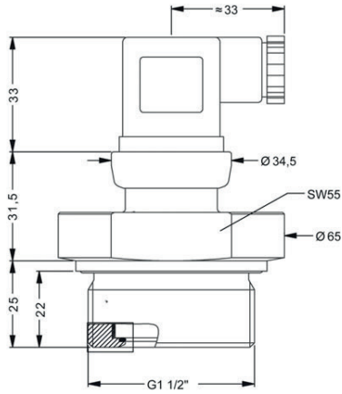
G1 1/2" EN 837
