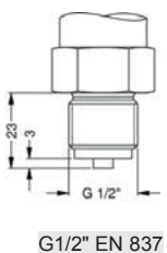
G1/2" EN 837
