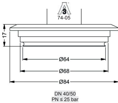
Varivent ®
