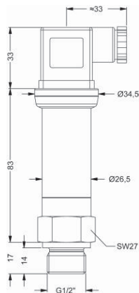
G1/2" DIN 3852
