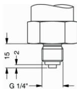
G1/4" EN 837
