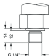
G1/4" DIN 3852
