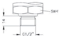
G1/2" DIN 3852
