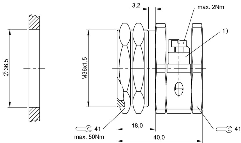
1) Зажимная скоба
