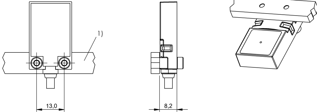
1) Крепежная пластина
