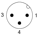
II Конт. 1: коричневый Конт. 3: синий Конт. 4: черный
