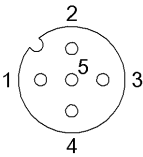
I Конт. 1: коричневый Конт. 2: белый Конт. 3: синий Конт. 4: черный Конт. 5: не занят
