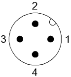
II Конт. 1: коричневый Конт. 2: белый Конт. 3: синий Конт. 4: черный
