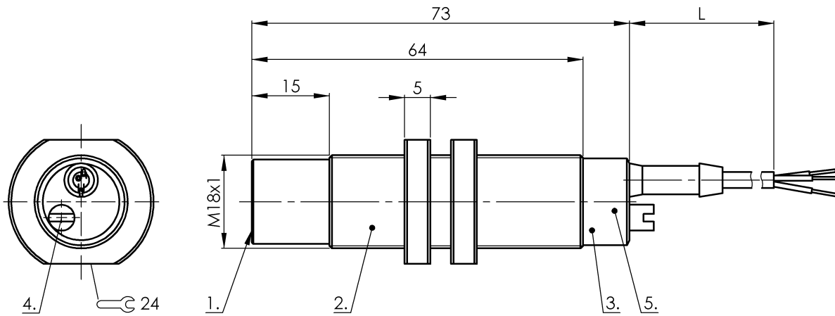
1) Активная поверхность 2) Корпус 3) Крышка 4) Потенциометр 5) Функциональный СИД
