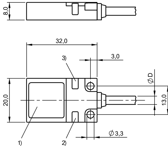
1) Активная поверхность 2) СИД зеленый 3) СИД желтый
