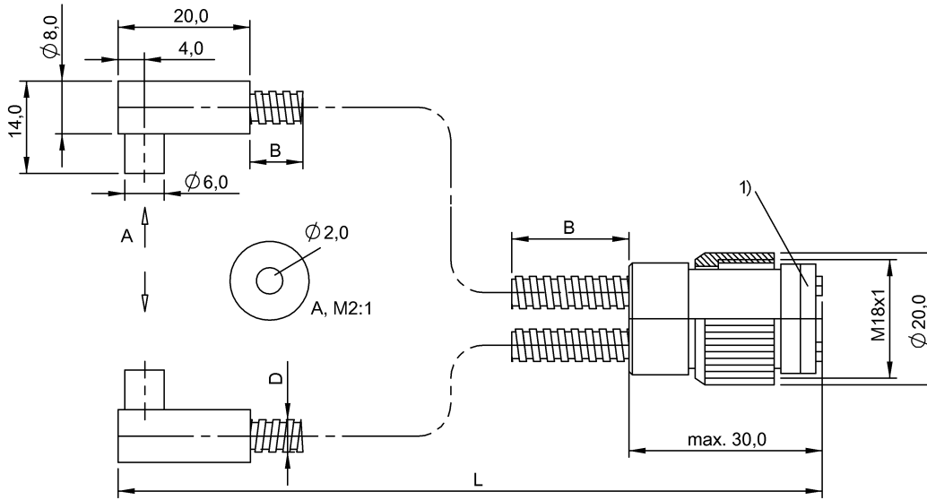
1) Съёмная шайба
