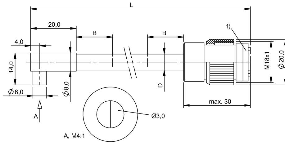
1) Съемная шайба
