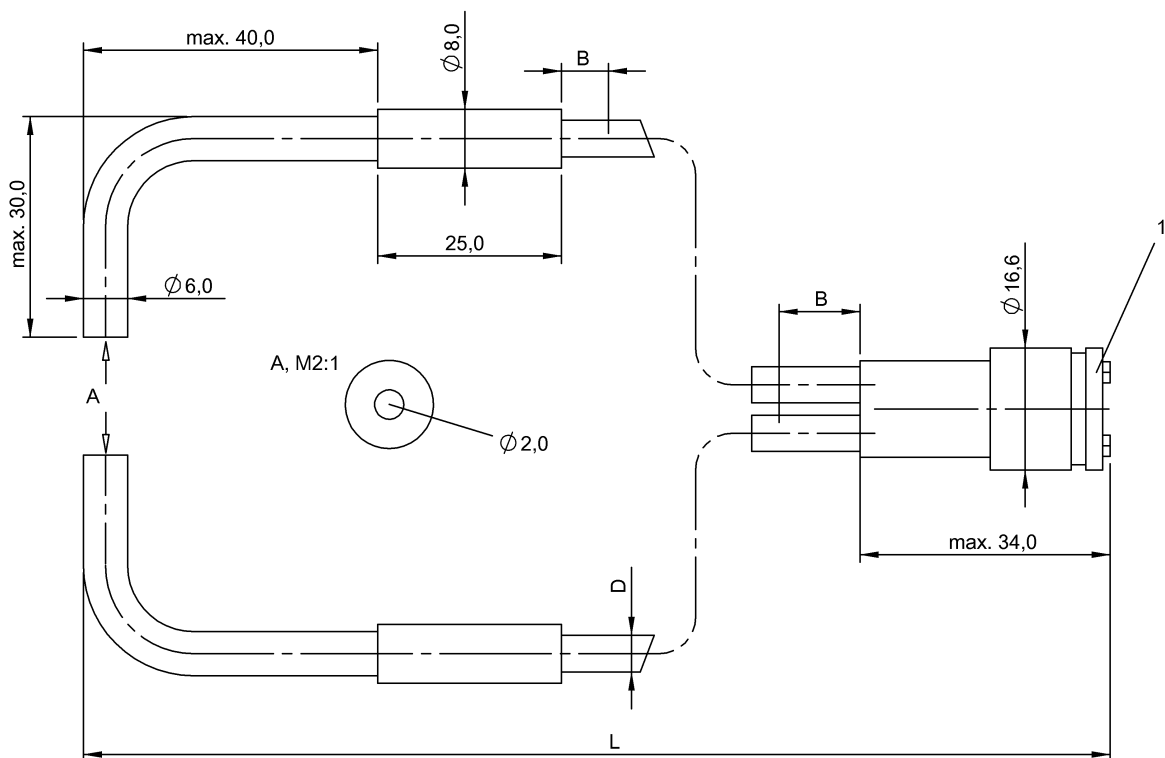
1) Съемная шайба
