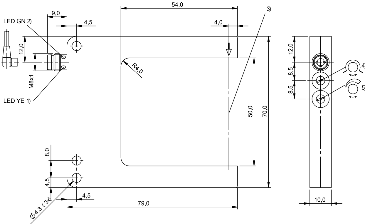
1) Функция выхода 2) Напряжение питания 3) Оптическая ось 4) Включение при освещении / затемнении 5) Чувствительность
