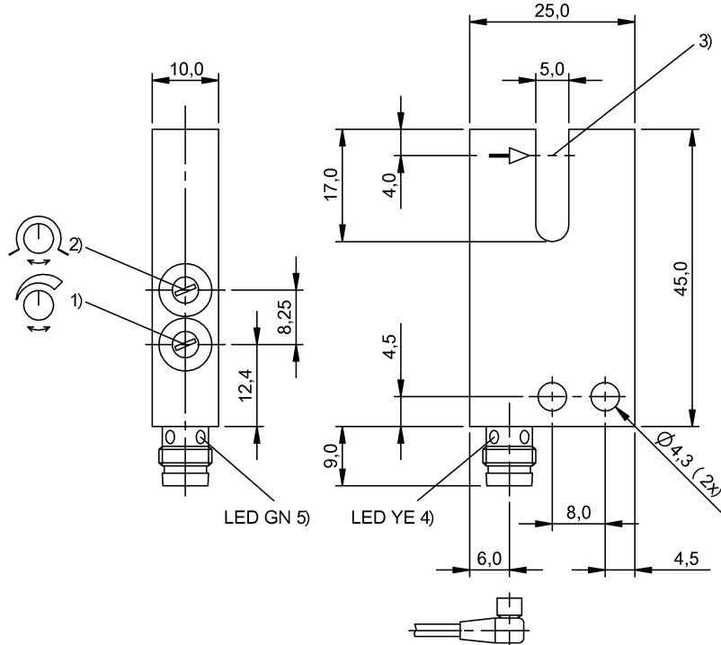
1) Чувствительность 2) Включение при освещении / затемнении 3) Оптическая ось 4) Функция выхода 5) Напряжение питания
