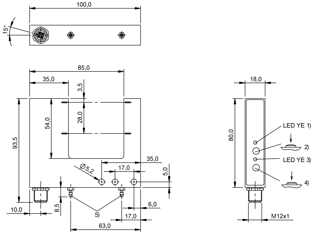
1) Q1 активен / сбой 2) Q1: чувств., светло/темно 3) Q2 активен / сбой 4) Q2: чувств., светло/темно 5) Пневматический разъем PK-3
