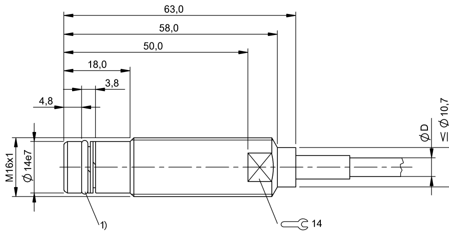
1) Упл. кольцо с опорным кольцом
