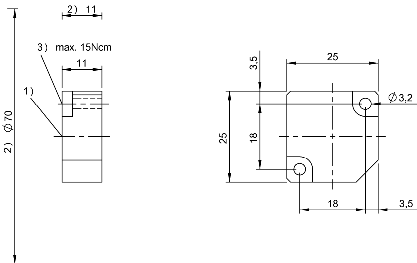
1) Активная поверхность 2) Свободная зона 3) Момент затяжки
