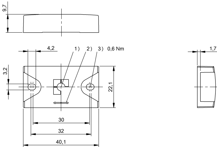
1) Активная поверхность 2) Ось записи / считывания 3) Момент затяжки
