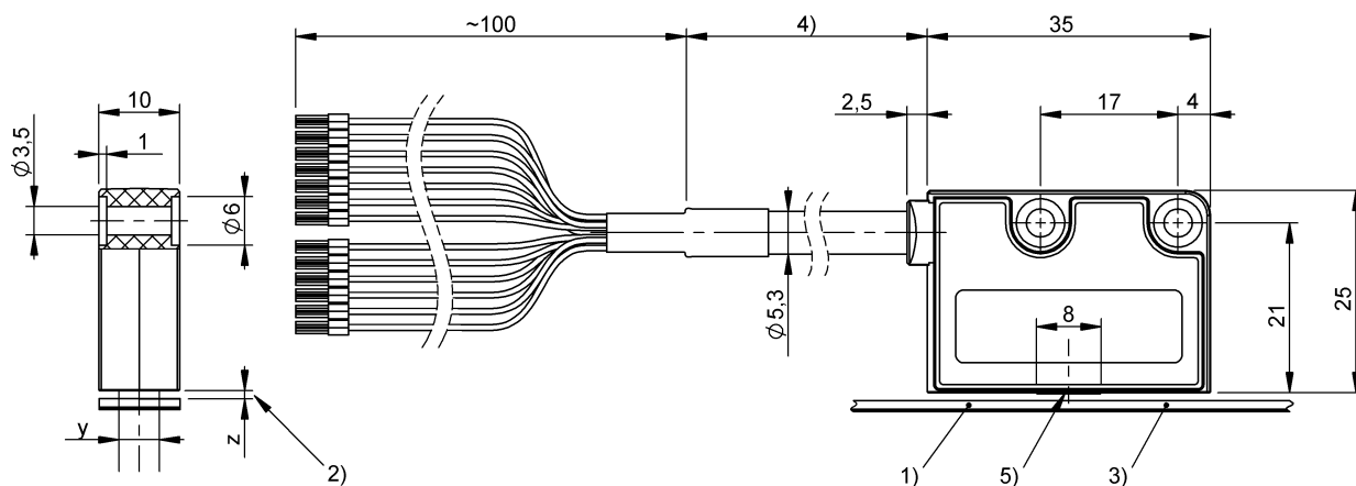
1) Не входит в комплект поставки 2) Расстояние до мерной ленты 3) Мерный объект 4) Длина кабеля 5) активная измер. поверхность
